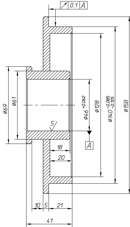
Рис. 41. Кондуктор
