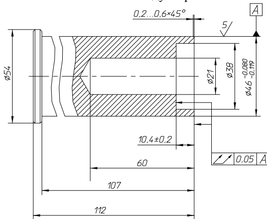
Рис. 42. Оправка
