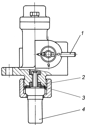
Рис. 19. Включатель муфты привода вентилятора:
