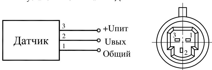
Рис. 29. Принципиальная электрическая схема подключения датчика
