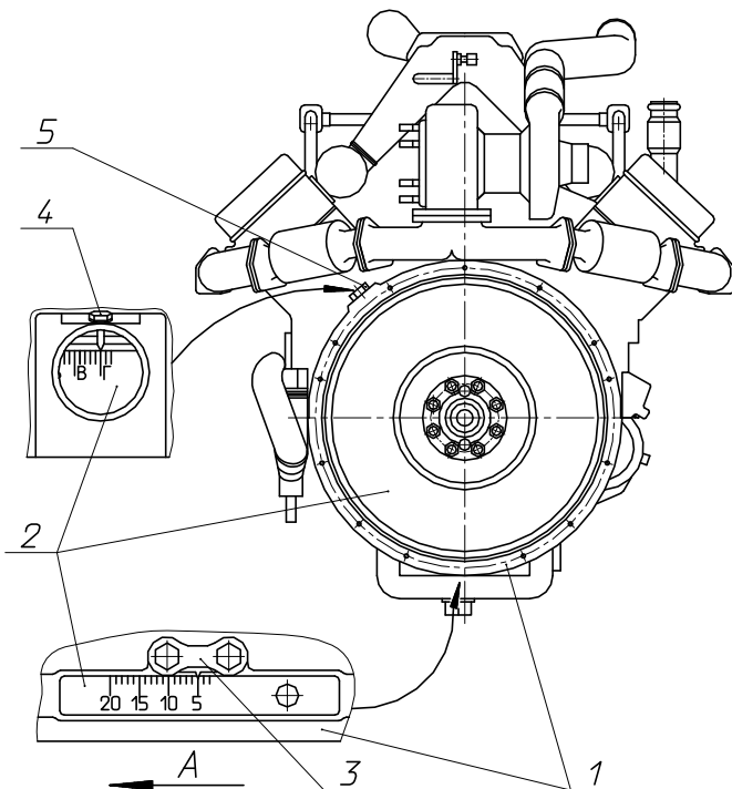
Рис. 17. Совмещение меток на маховике с указателями картера маховика:
