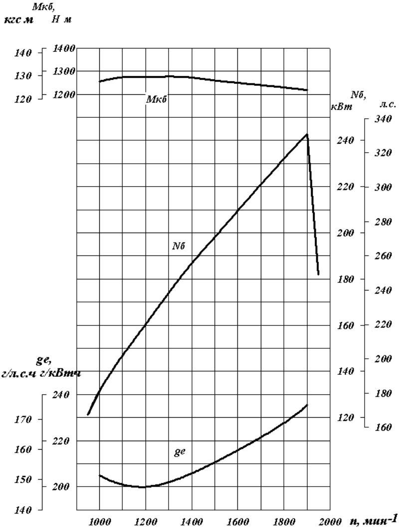
Рис. 1. Скоростная характеристика двигателя ЯМЗ-6582.10
