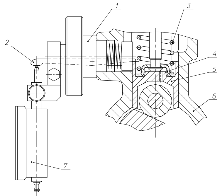
Рис. 15. Измерение величины подъема толкателя:
