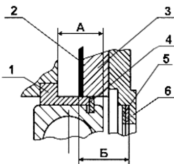
Рисунок 28 – Регулировка осевого люфта вторичного вала:
