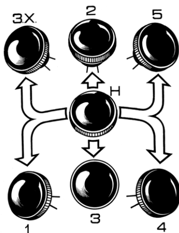
Рис. 29. Схема положений рычага передач ЯМЗ-236Н
