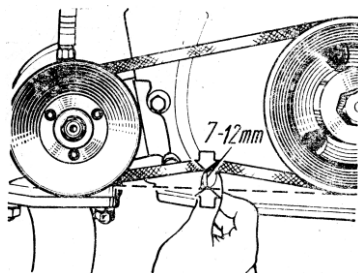
Рис. 8. Проверка натяжения ремня привода водяного насоса
