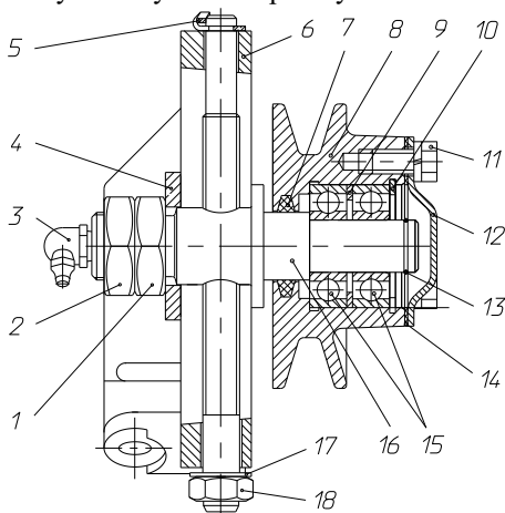
Рис. 12. Натяжное устройство компрессора:
