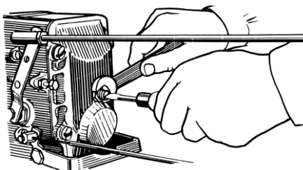
Рис. 20. Вывертывание корпуса буферной пружины
