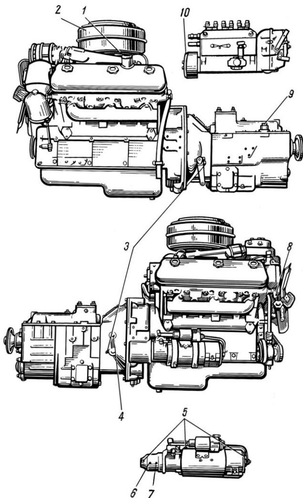
Рис. 2. Точки смазки
