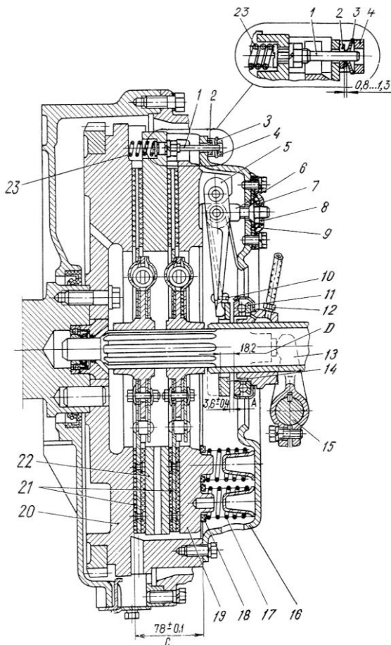
Рис. 26. Сцепление ЯМЗ - 238:
