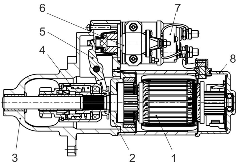
Рисунок 42 – Стартер 5432.3708-01:
