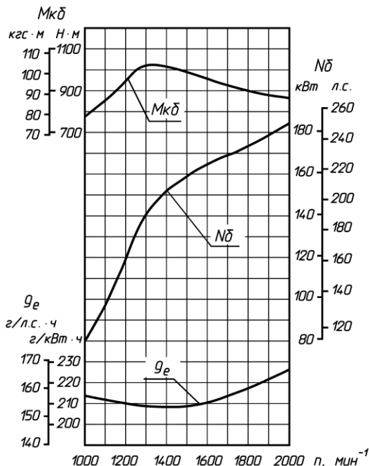
Рис. 6. Скоростная характеристика двигателя ЯМЗ-236БЕ: Mkб. - крутящий момент брутто; Nб - номинальная мощность брутто; ge-удельный расход топлива; n - частота вращения коленчатого вала
