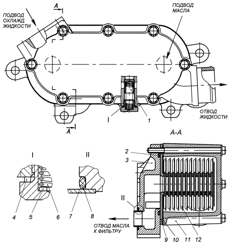
Рис. 49. Жидкостно-масляный теплообменник:
