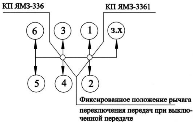
Рис. 28. Схема переключения передач КП.
