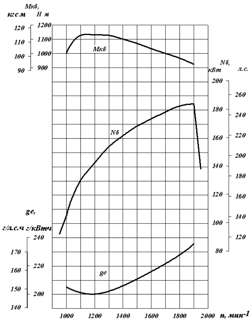
Рис. 1. Скоростная характеристика двигателя ЯМЗ-6562.10
