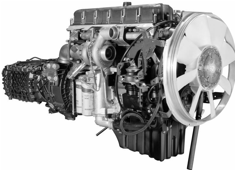
Рис. 1.1. Силовой агрегат ЯМЗ-6501 – вид справа
