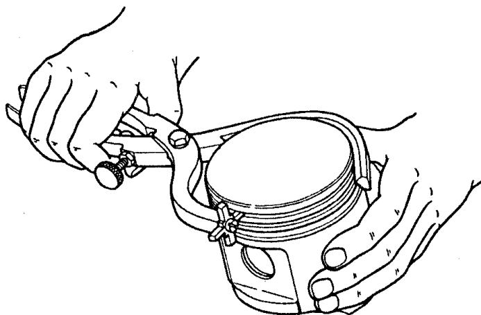
Рис.56. Очистка канавок поршневых колец от нагара с помощью приспособления 5-У-27691
