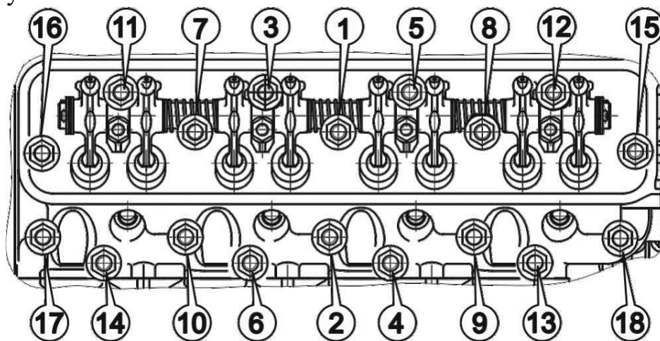
Рис.14. Порядок подтяжки гаек крепления головок цилиндров
