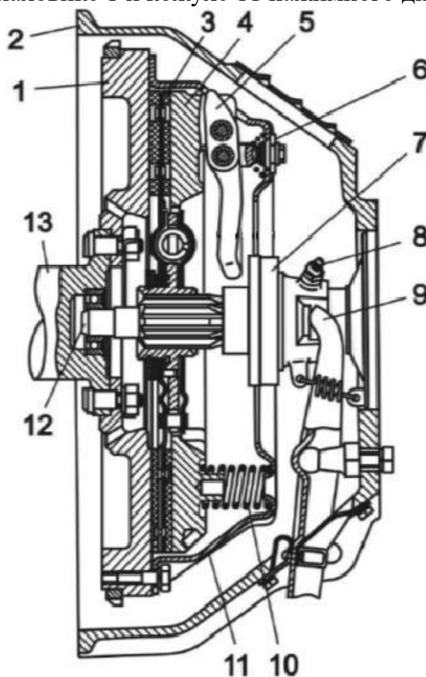
Рис.49. Сцепление:
