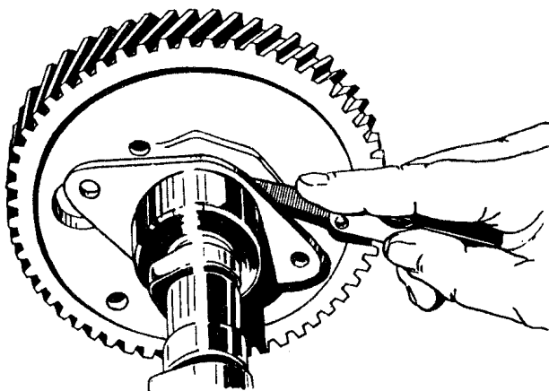
Рис.74. Проверка осевого зазора распределительного вала
