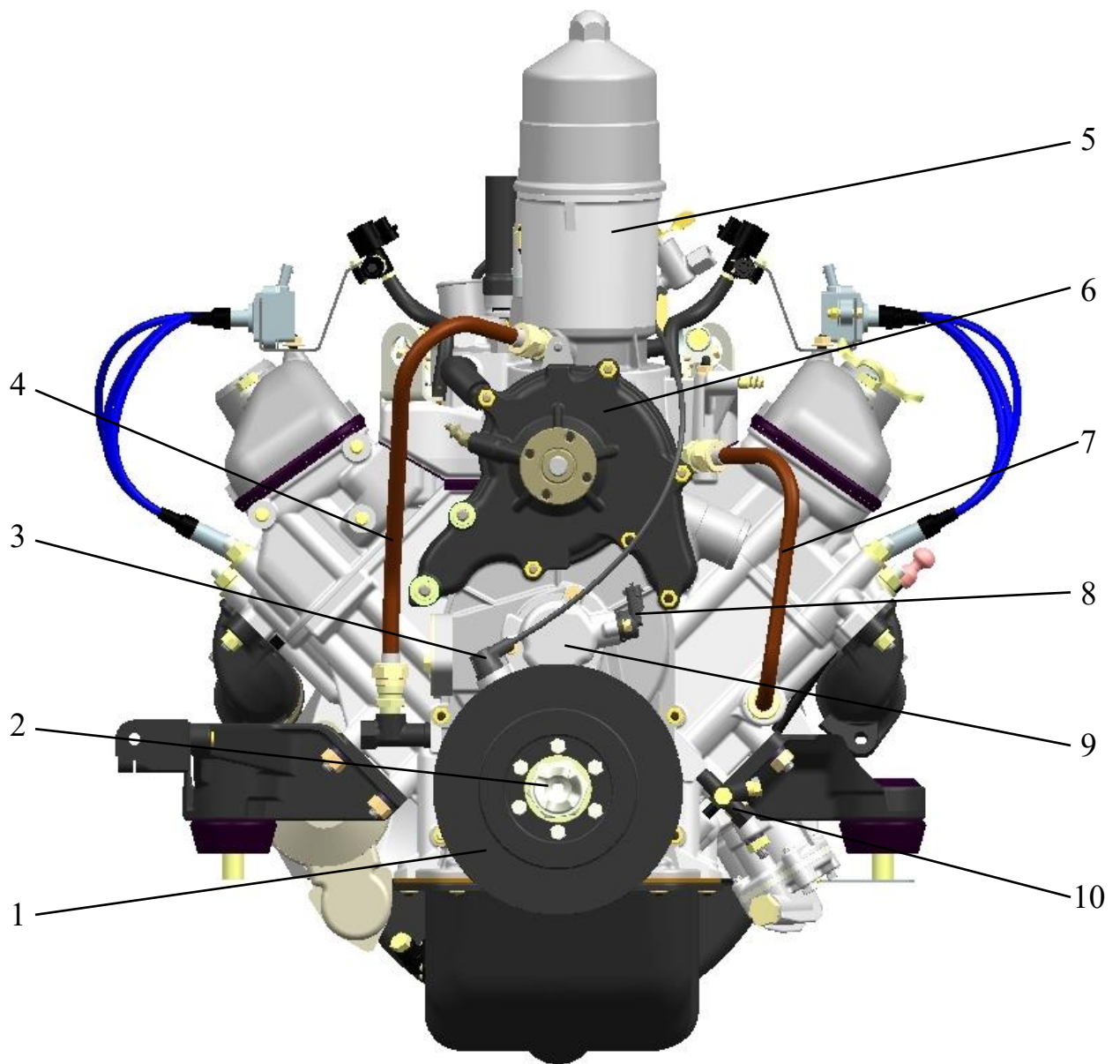
Рис.2 Вид двигателя спереди (комплектация с газовым оборудованием):
