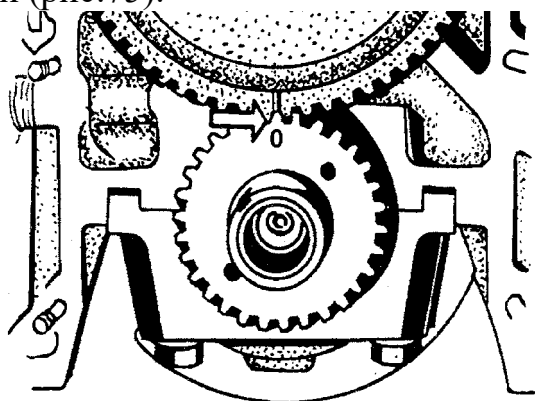
Рис.75. Установка шестерен распределения:
