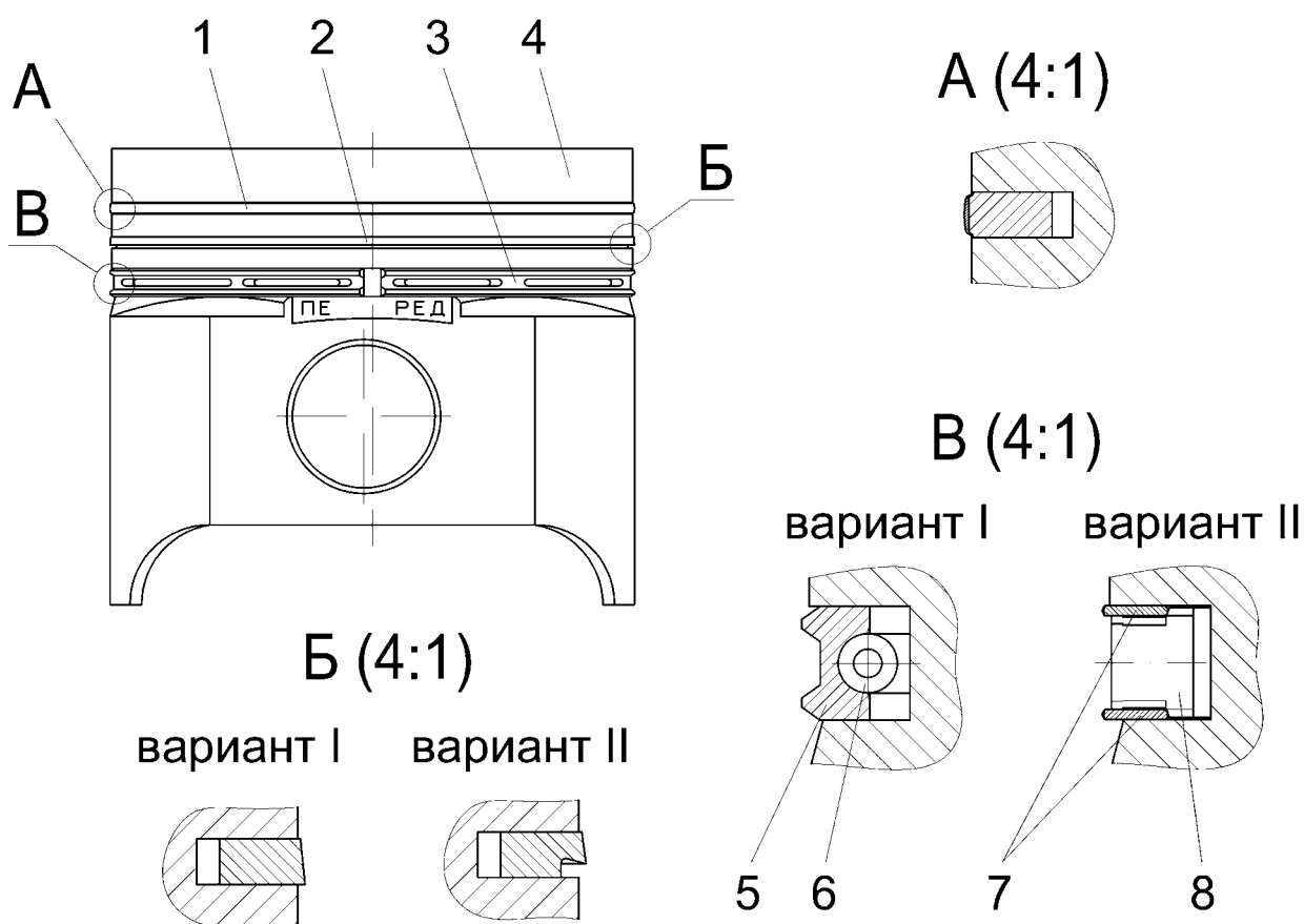
Рис.11. Поршневые кольца:
