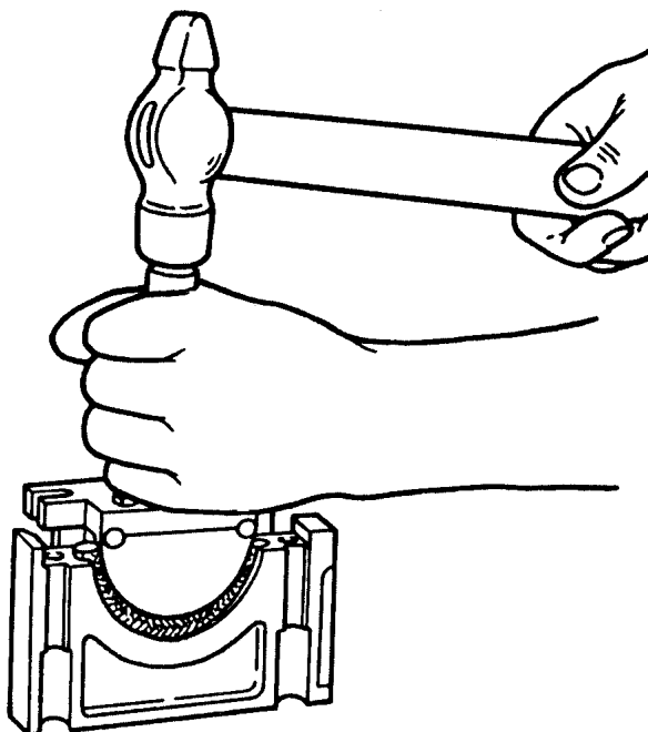
Рис.66. Установка сальниковой набивки в держатель сальника
