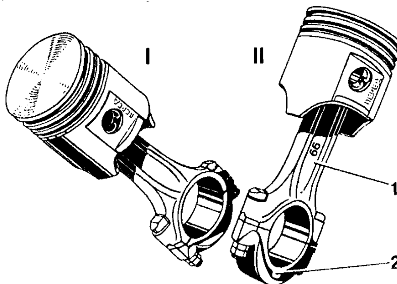
Рис.72. Соединение шатуна с поршнем:
