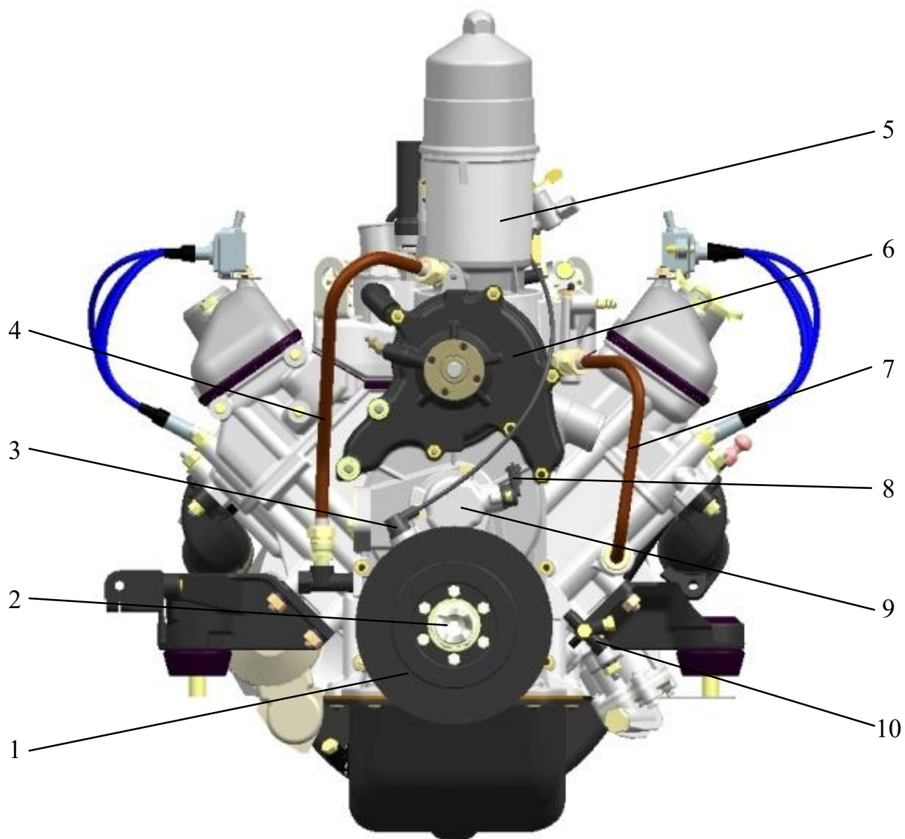
Рис.6. Вид двигателя спереди (бензиновая комплектация):
