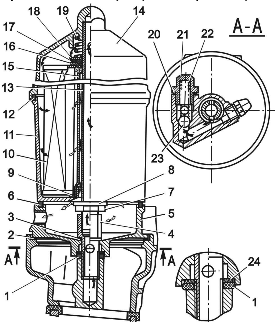
Рис.22. Масляный фильтр:
