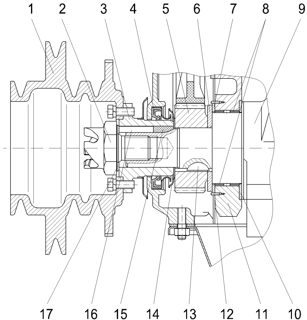
Рис.12. Передний конец коленчатого вала:
