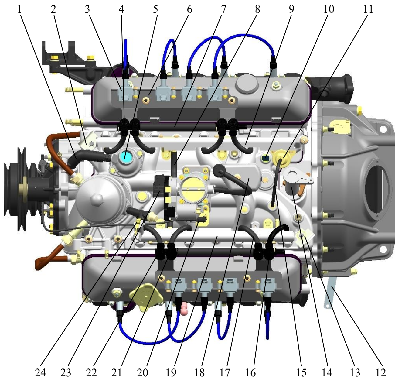
Рис.5. Вид сверху (комплектация с газовым оборудованием):
