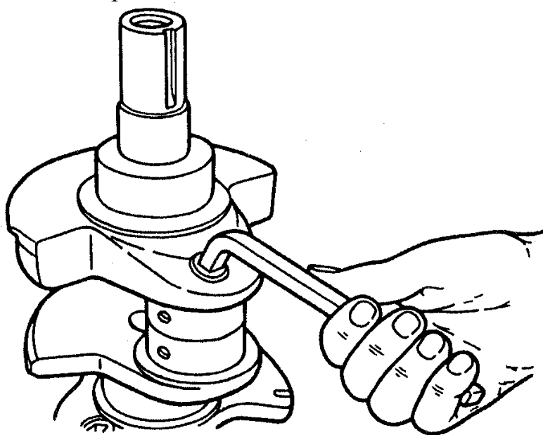
Рис.57. Вывертывание пробок грязеуловителей из коленчатого вала
