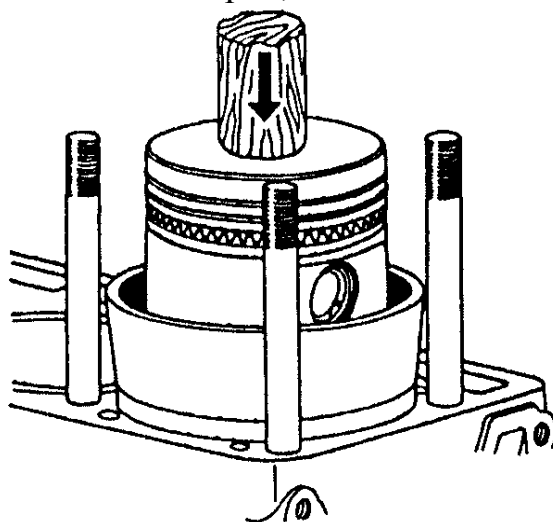
Рис.73. Установка поршня с кольцами в цилиндр
