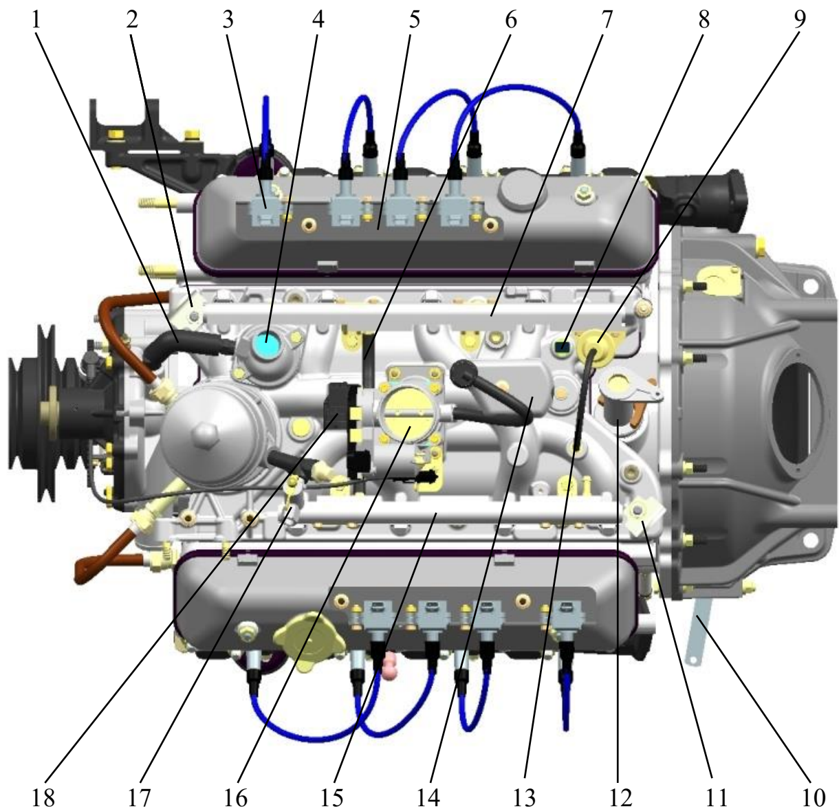
Рис.7. Вид двигателя сверху (бензиновая комплектация):
