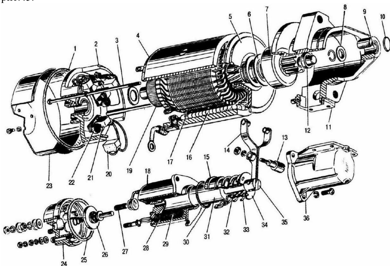
Рис.45. Устройство стартера СТ230А1:
