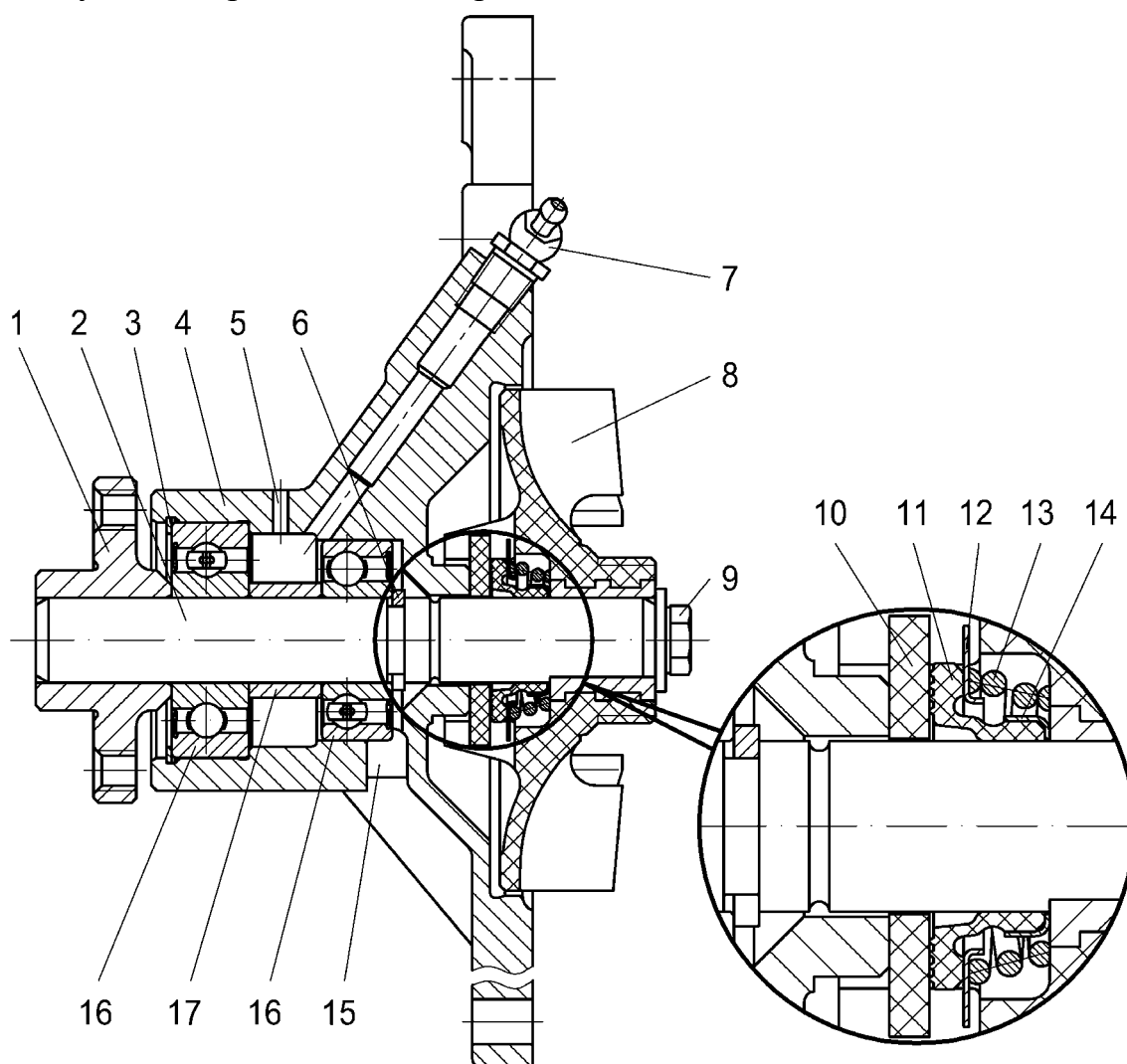
Рис.26. Водяной насос с уплотнением старого образца:
