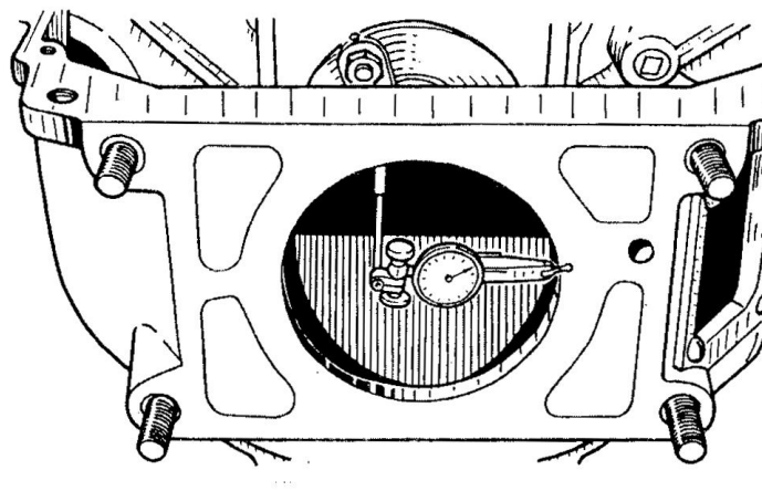
Рис.51. Проверка перпендикулярности заднего торца картера сцепления к оси коленчатого вала
