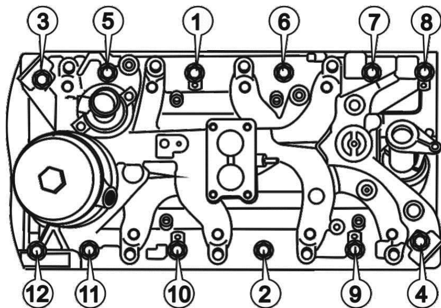
Рис.15. Порядок подтяжки гаек крепления впускной трубы
