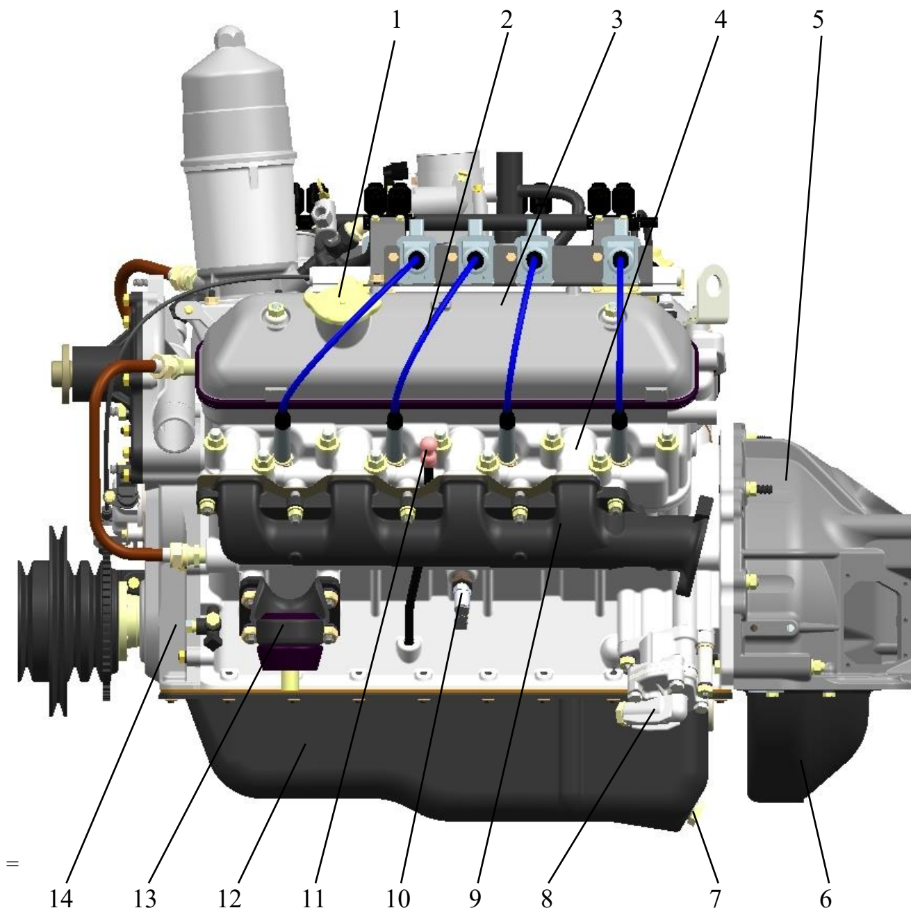
Рис.4. Вид двигателя слева (комплектация с газовым оборудованием):
