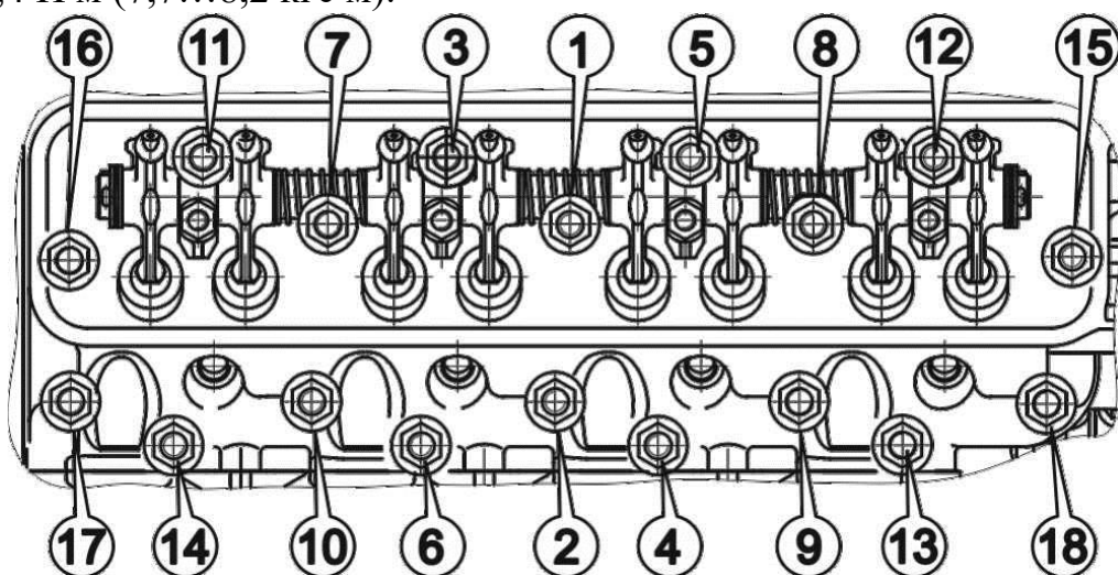
Рис.77. Порядок затяжки гаек головки цилиндров
