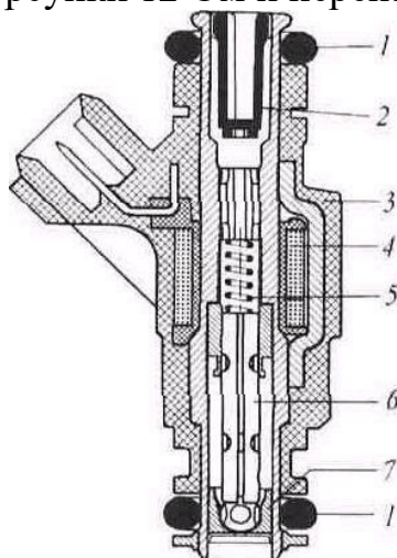
Рис.32. Электромагнитная форсунка:
