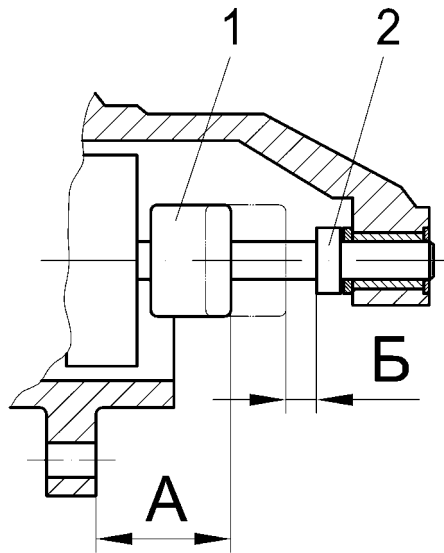
Рис.48. Схема регулировки:
