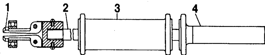
Рис.55. Съемник 7823-6090 для выпрессовки подшипника первичного вала коробки передач из коленчатого вала:
