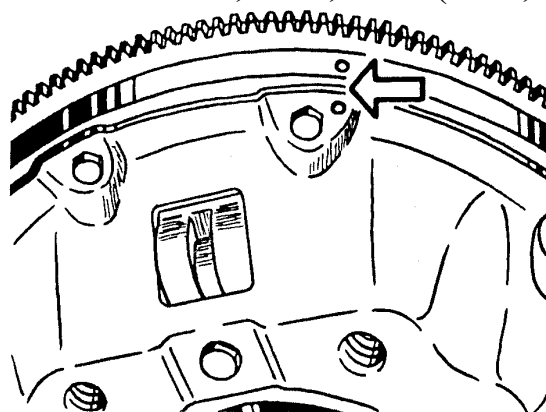
Рис.67. Расположение меток на маховике и кожухе сцепления
