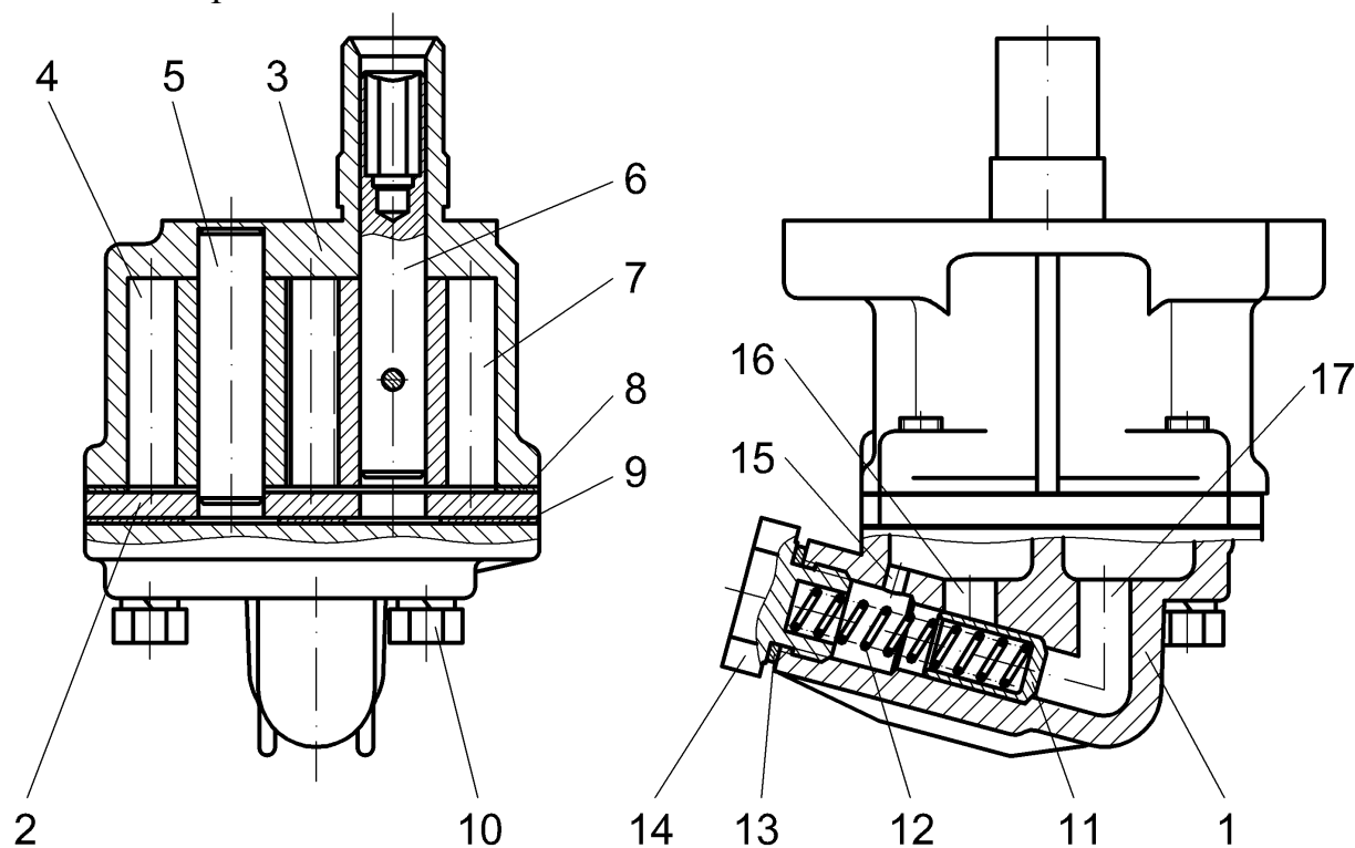
Рис.20. Масляный насос:
