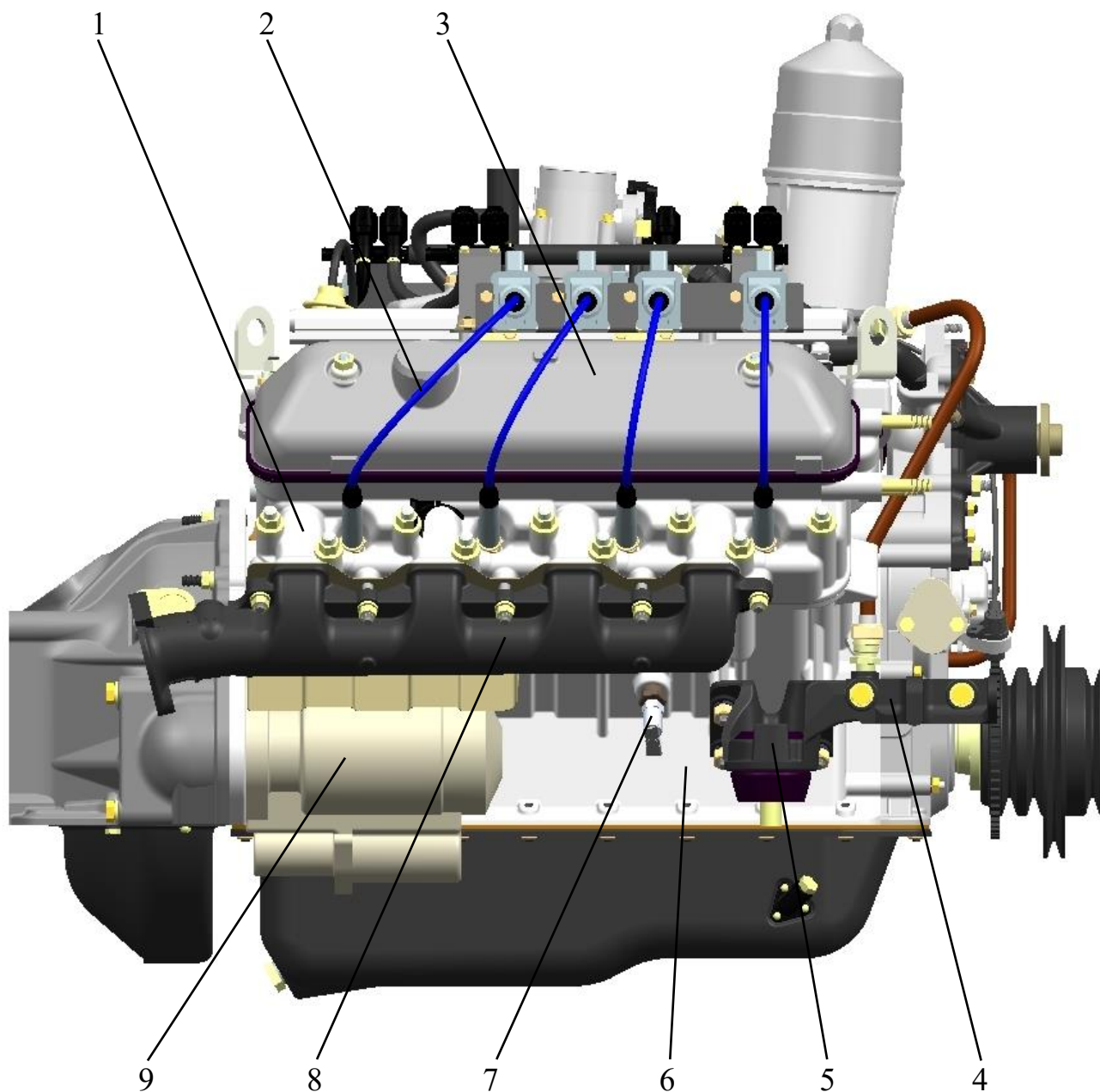
Рис.3. Вид двигателя справа (комплектация с газовым оборудованием):
