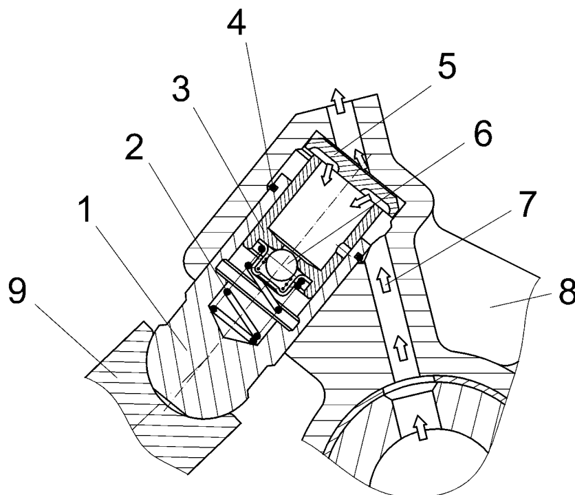
Рис.18. Гидрокомпенсатор:
