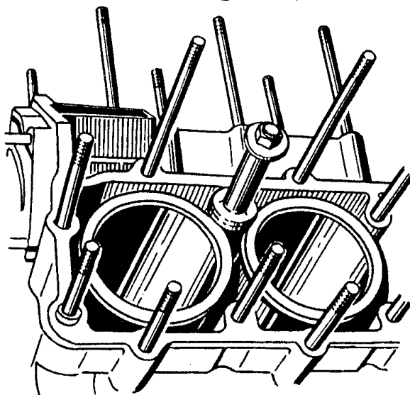
Рис.52. Закрепление гильз втулками - зажимами
