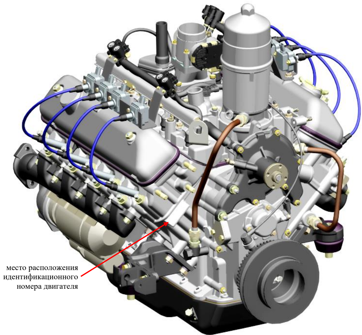
Рис.1. Общий вид двигателя (комплектация с газовым оборудованием)
