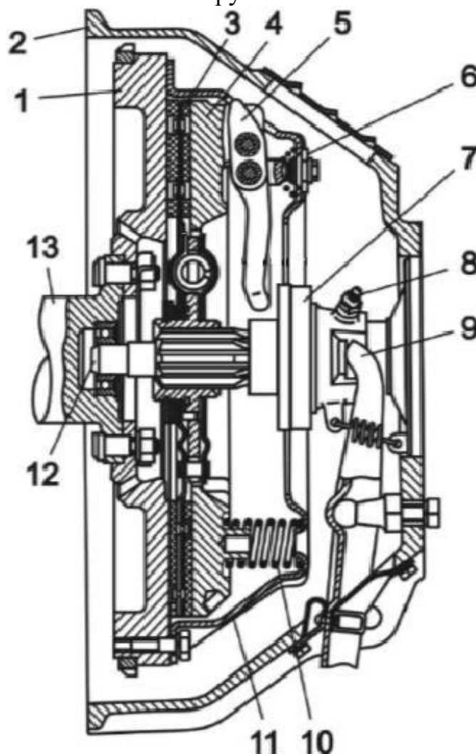
Рис.66. Сцепление:
