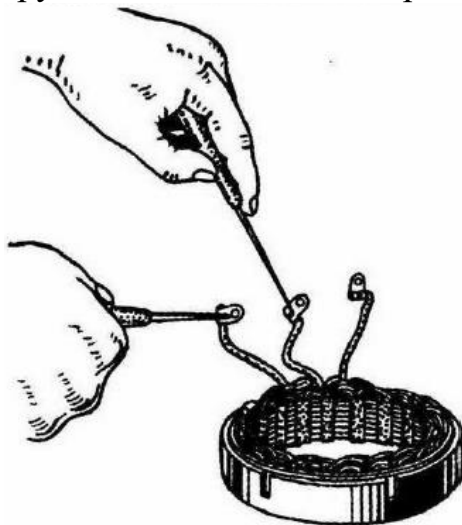
Рис.53. Проверка обмоток статора на отсутствие межвитковых замыканий
