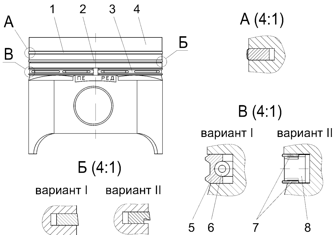
Рис.6. Поршневые кольца:
