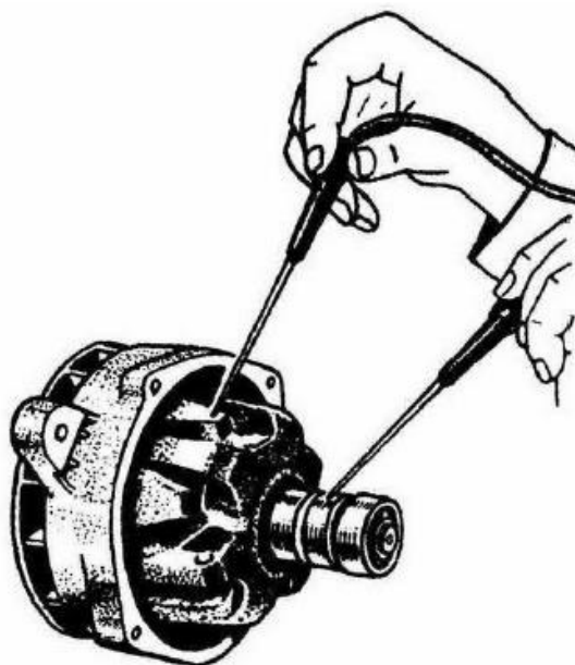
Рис.54. Проверка ротора на отсутствие замыкания обмотки на корпус
