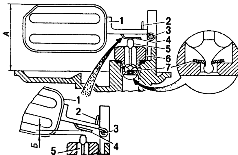
Рис.29. Поплавковый механизм карбюратора:
