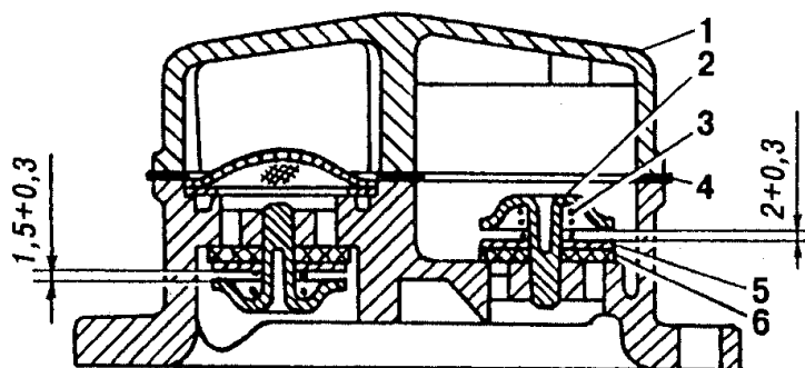
Рис.84. Головка бензинового насоса:
