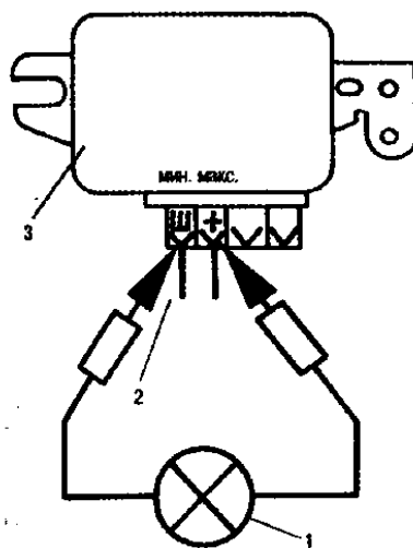
Рис.60. Схема проверки исправности регулятора напряжения:
