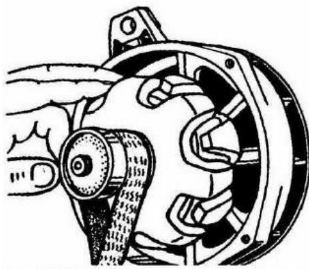
Рис.55. Зачистка контактных колец наждачной бумагой
