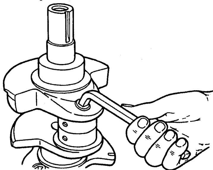
Рис.74. Выверачивание пробок грязеуловителей из коленчатого вала
