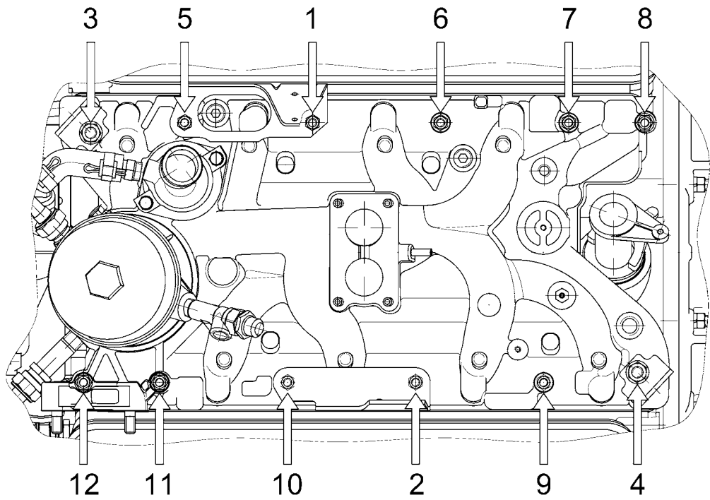
Рис.10. Порядок затяжки гаек впускной трубы
