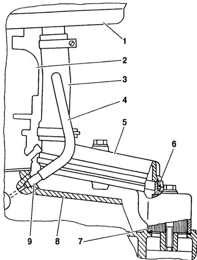
Рис.20. Схема системы вентиляции картера:
