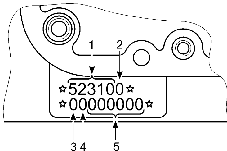
Рис.4. Идентификационный номер двигателя:
