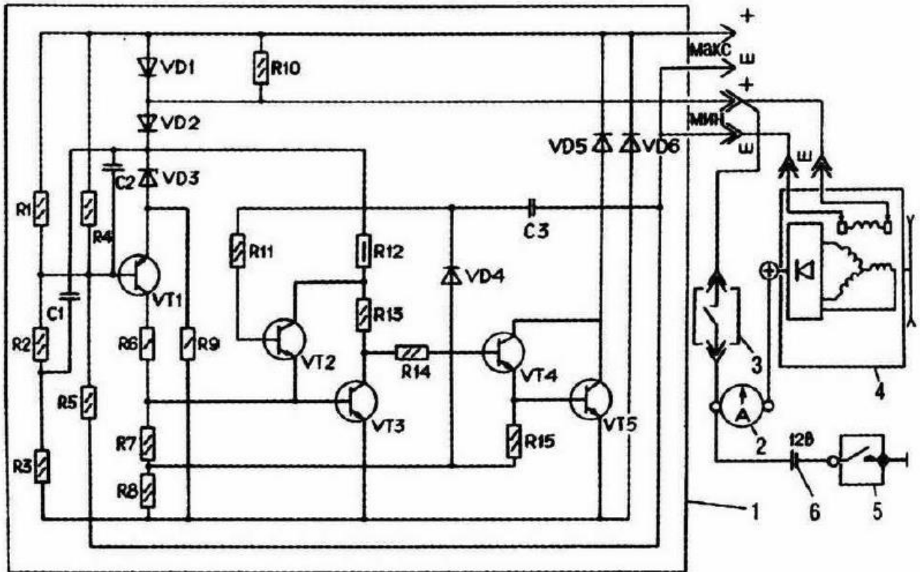
Рис.59. Электрическая схема регулятора напряжения 131.3702 и его соединения с генератором:
