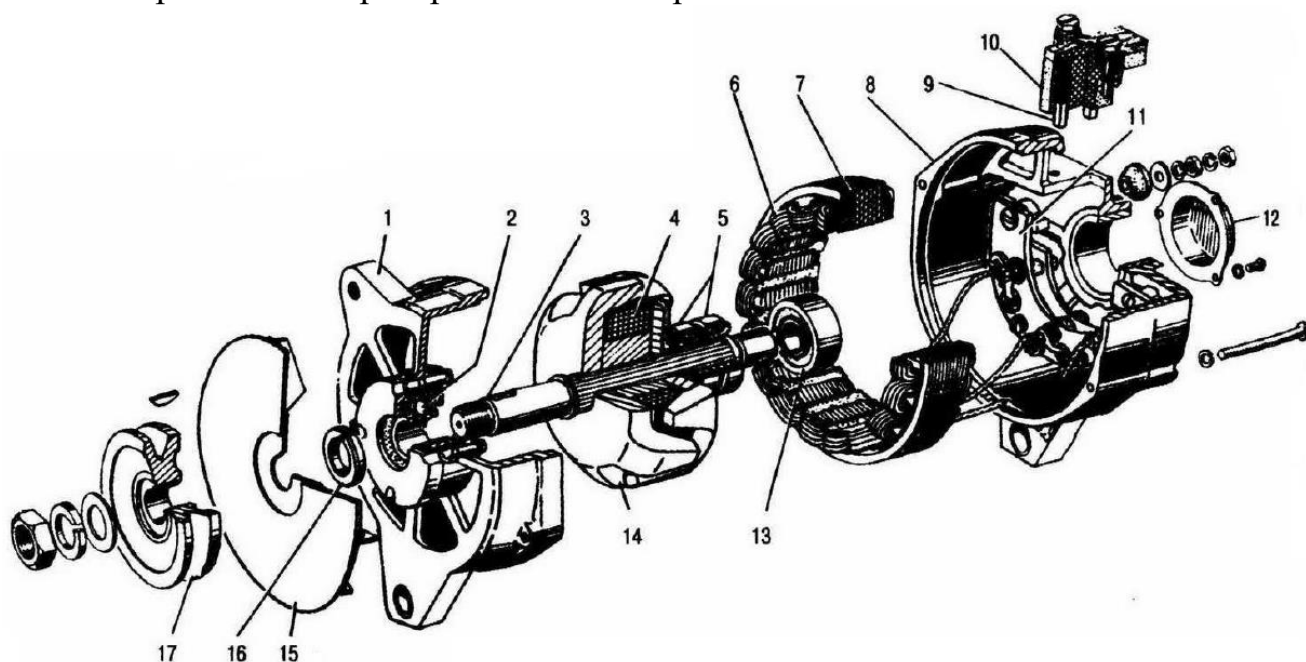
Рис.48. Генератор:
