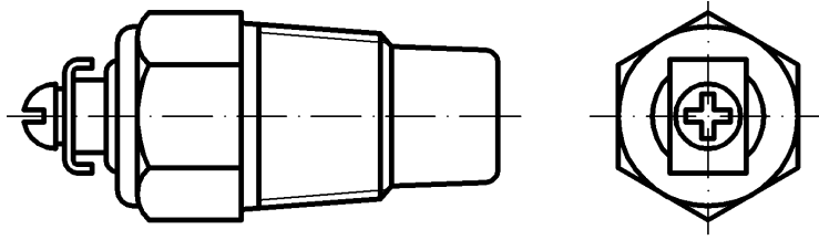
Рис.64. Датчик указателя температуры охлаждающей жидкости
