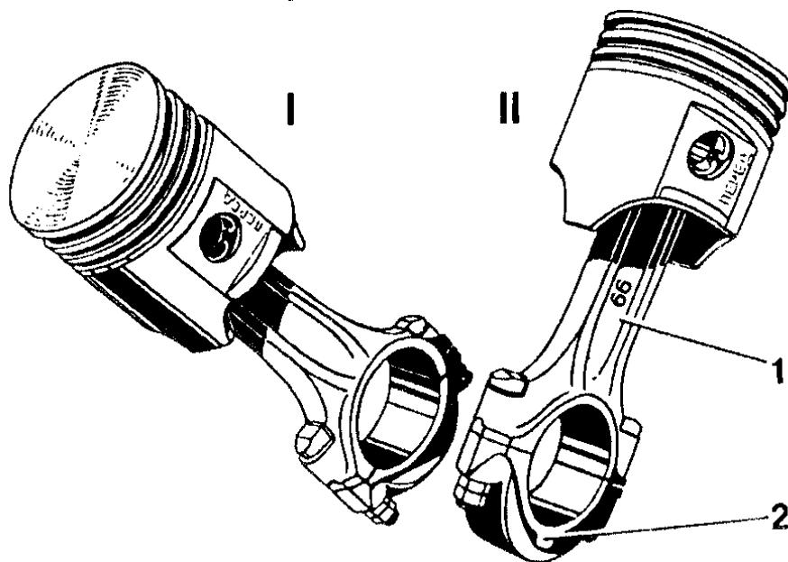
Рис.92. Соединение шатуна с поршнем:
