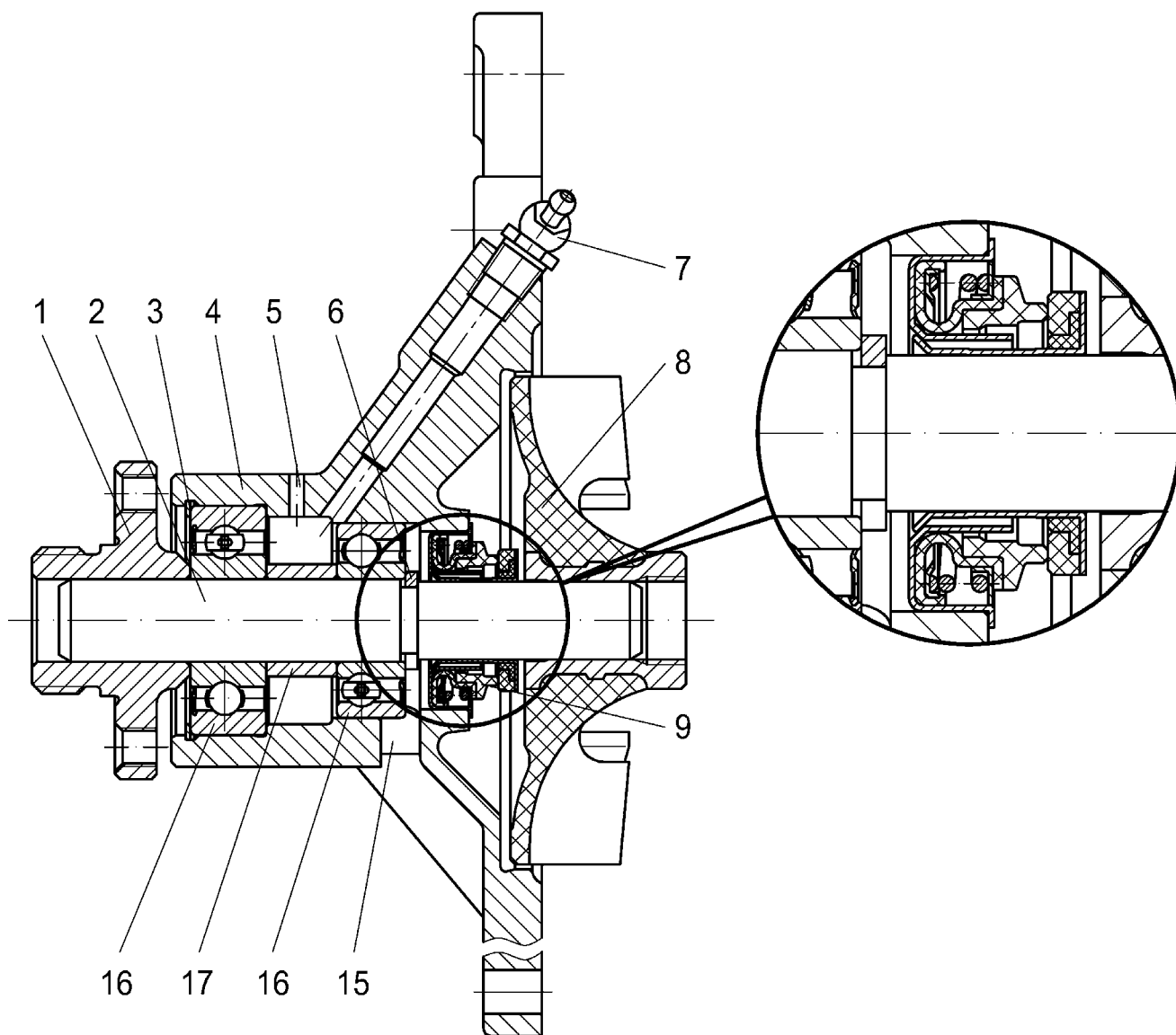
Рис.23. Водяной насос с уплотнением нового образца:
