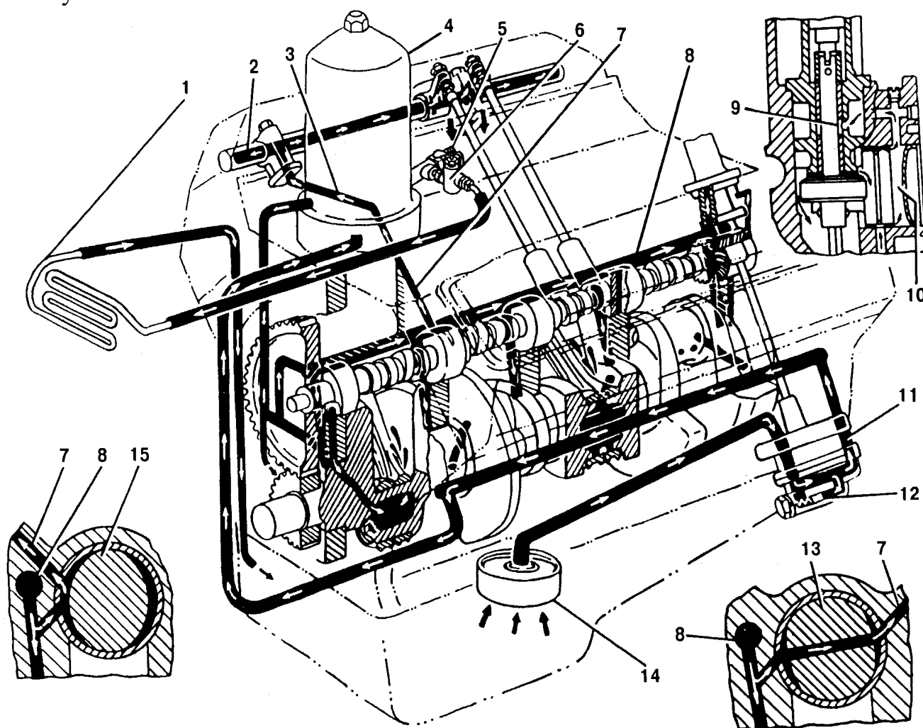
Рис.14. Схема смазки двигателя:
