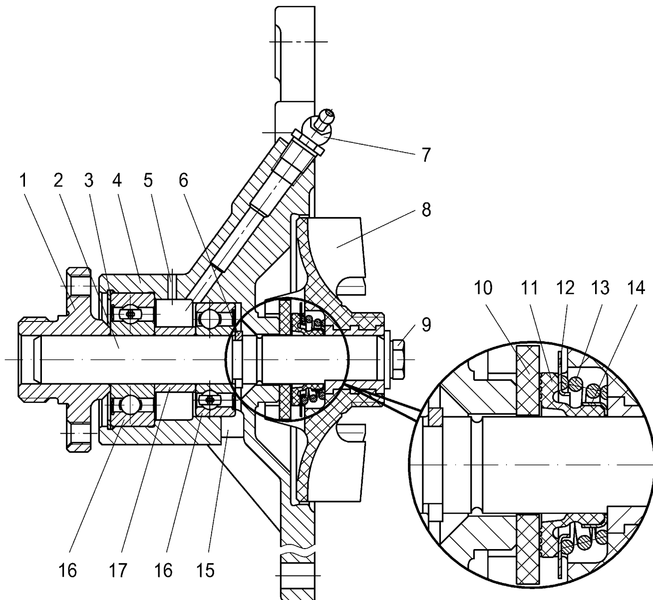
Рис.22. Водяной насос с уплотнением старого образца:
