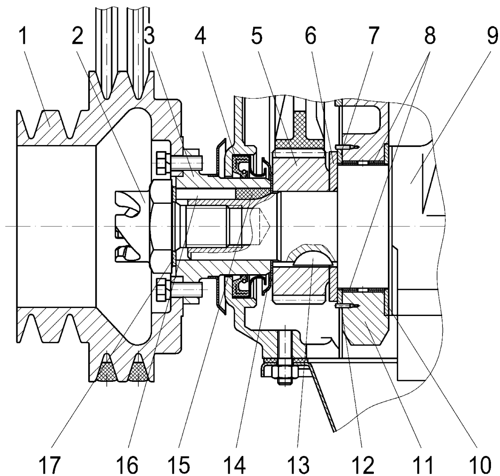
Рис.7. Передний конец коленчатого вала:
