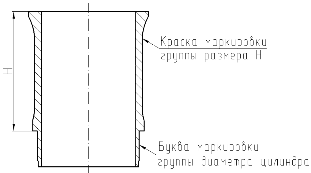
Рис.90. Маркировка гильзы цилиндра
