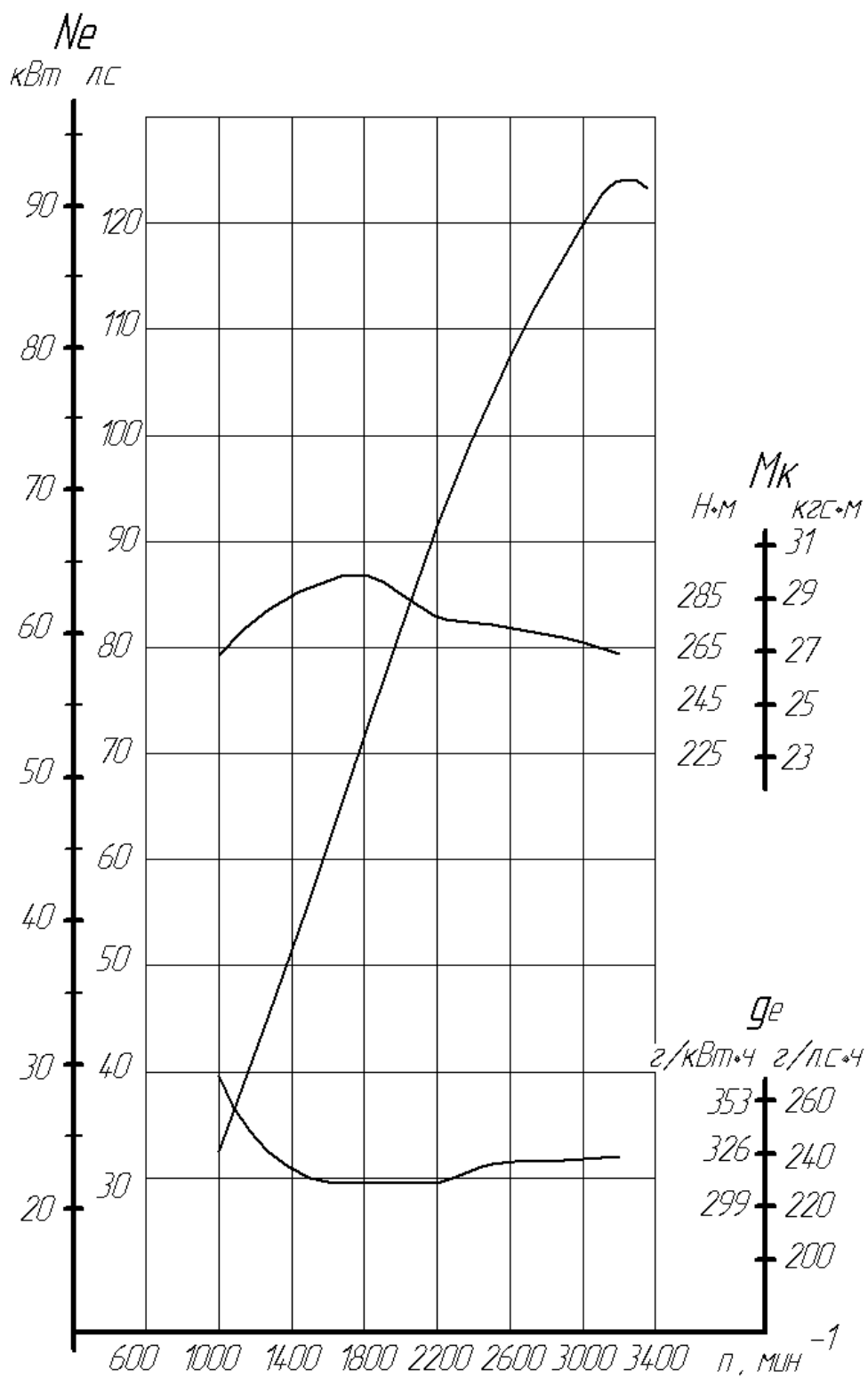
Рис.3. Внешняя скоростная характеристика двигателя
