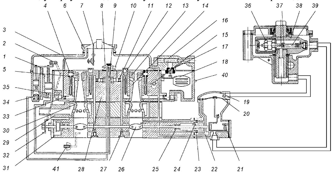
Рис.27. Схема карбюратора К135Г и датчика-ограничителя частоты вращения:
