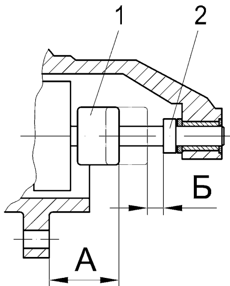
Рис.47. Схема регулировки:
