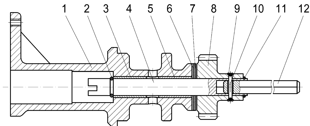
Рис.16. Привод датчика-распределителя зажигания и масляного насоса:
