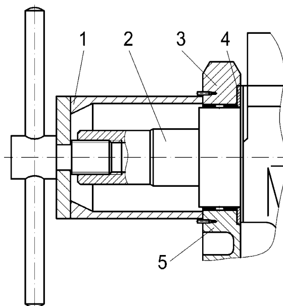
Рис.88. Установка крышки первой коренной опоры с оправкой:
