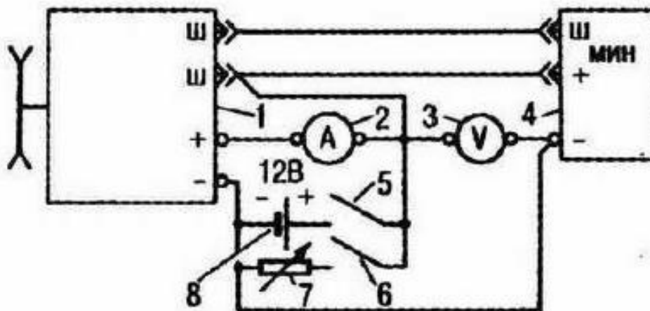
Рис.61. Схема проверки регулятора напряжения на стенде:
