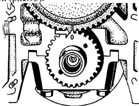
Рис.95. Установка шестерен распределения:
