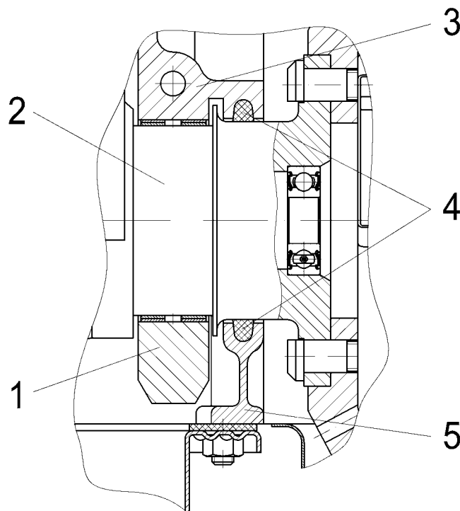
Рис.8. Задний конец коленчатого вала:
