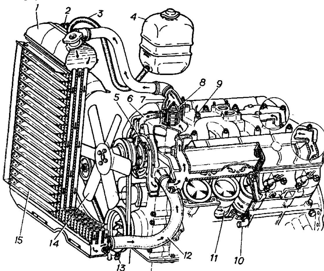
Рис.21. Система охлаждения:
