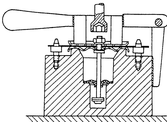
Рис.83. Приспособление для сборки диафрагмы
