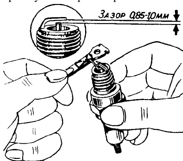
Рис.41. Регулировка зазора между электродами свечи зажигания
