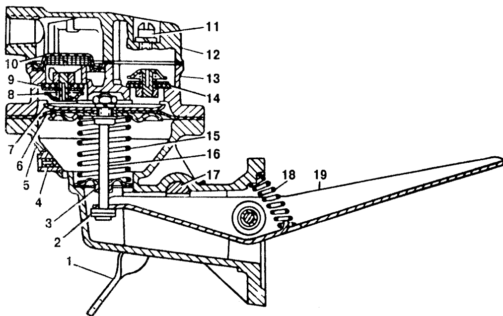
Рис.25. Бензиновый насос:
