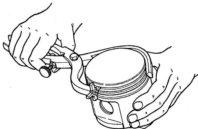
Рис.73. Очистка канавок поршневых колец от нагара с помощью приспособления 5-У-27691
