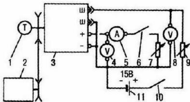
Рис.58. Схема проверки генератора на стенде:
