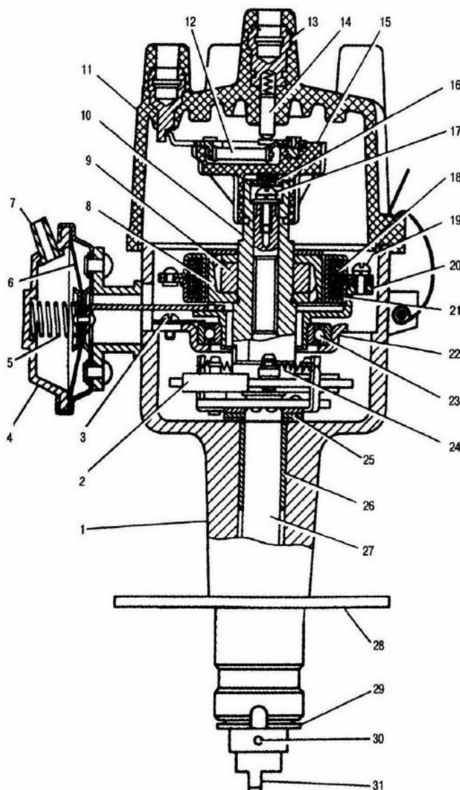
Рис.38. Датчик-распределитель зажигания:
