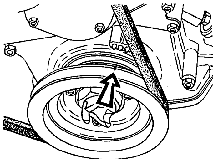
Рис.99. Установка поршня в ВМТ в первом цилиндре
