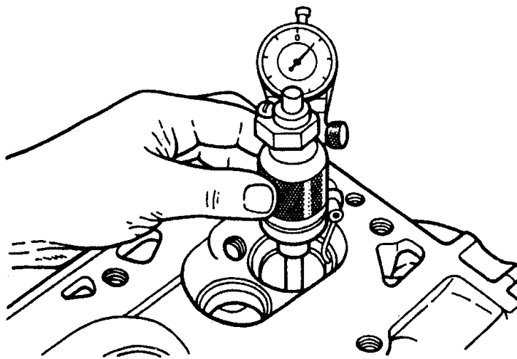
Рис.77. Измерение концентричности седла клапана относительно оси направляющей втулки
