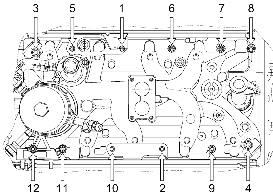
Рис.98. Порядок затяжки гаек впускной трубы
