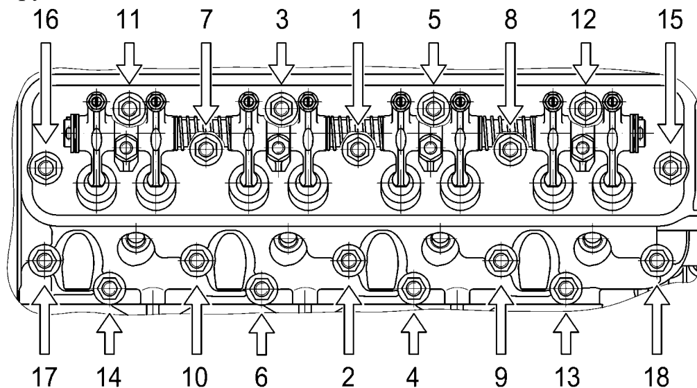
Рис.9. Порядок подтяжки гаек крепления головок цилиндров
