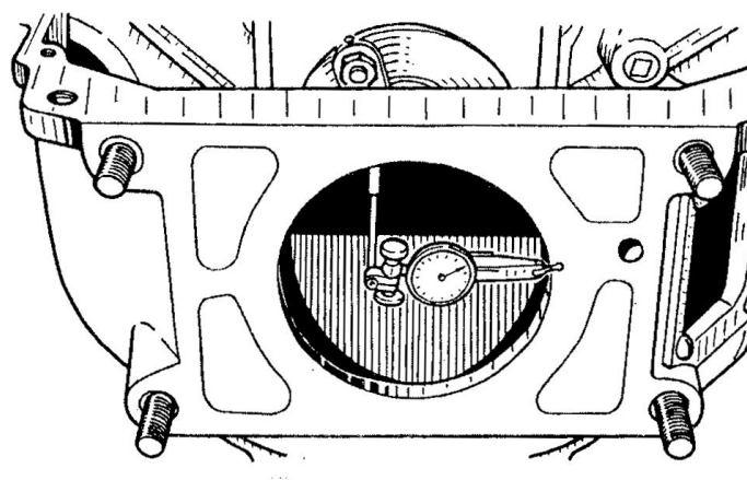
Рис.68. Проверка перпендикулярности заднего торца картера сцепления к оси коленчатого вала
