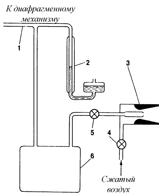
Рис.35. Схема проверки герметичности диафрагменного исполнительного механизма:
