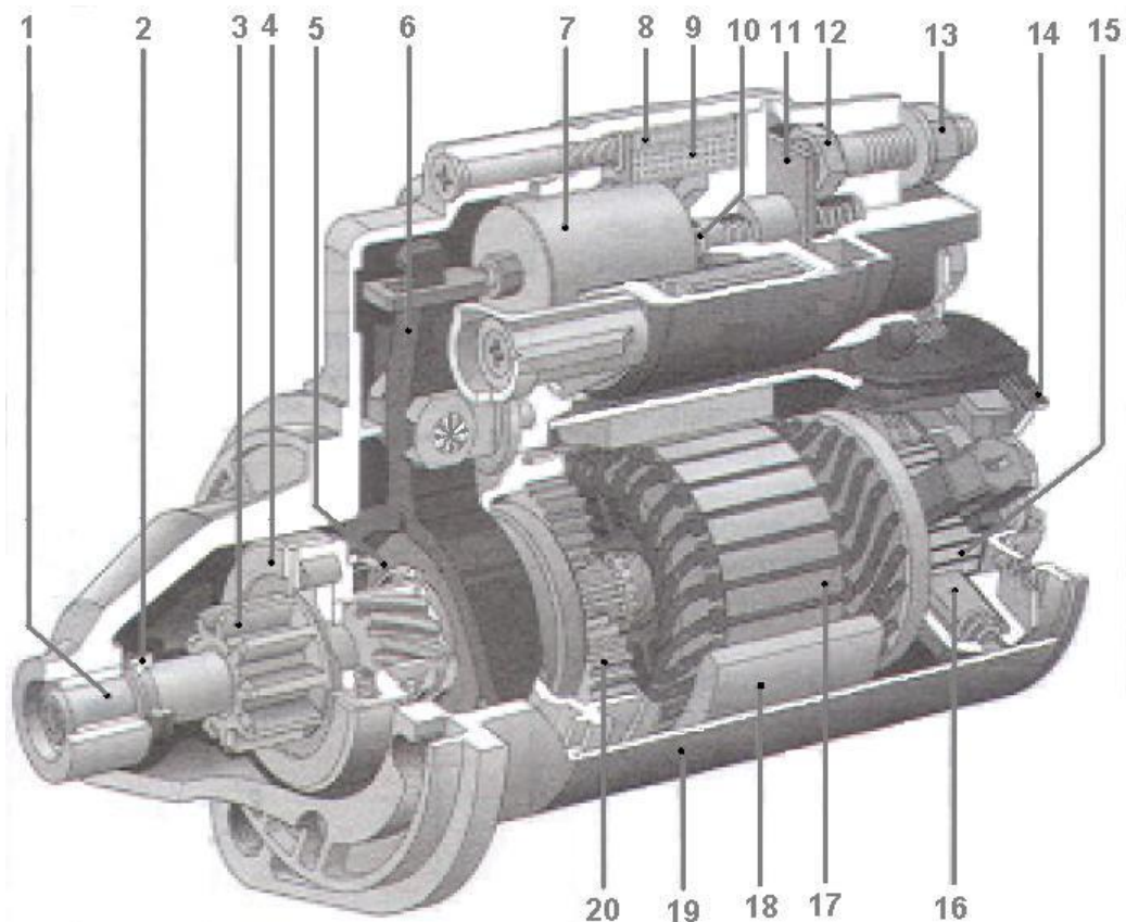
Рис.45. Устройство стартера 5234.3708:
