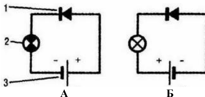
Рис.57. Схема проверки диодов с помощью контрольной лампы
