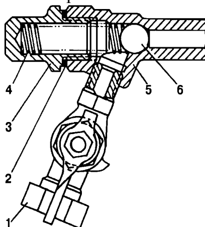
Рис.18. Предохранительный клапан и краник масляного радиатора:
