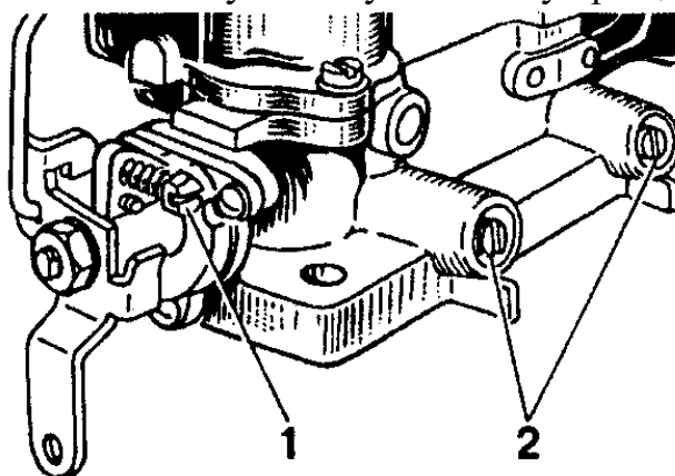
Рис.32. Регулировочные винты карбюратора:
