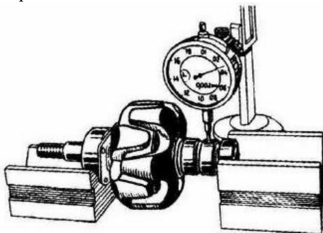
Рис.56. Проверка биения контактных колец
