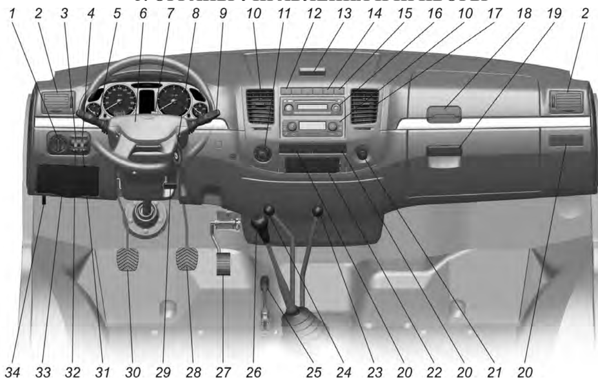
Рис. 5.1. Панель приборов и органы управления
