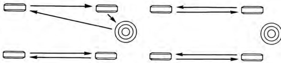
Рис. 9.11. Схема перестановки колес
