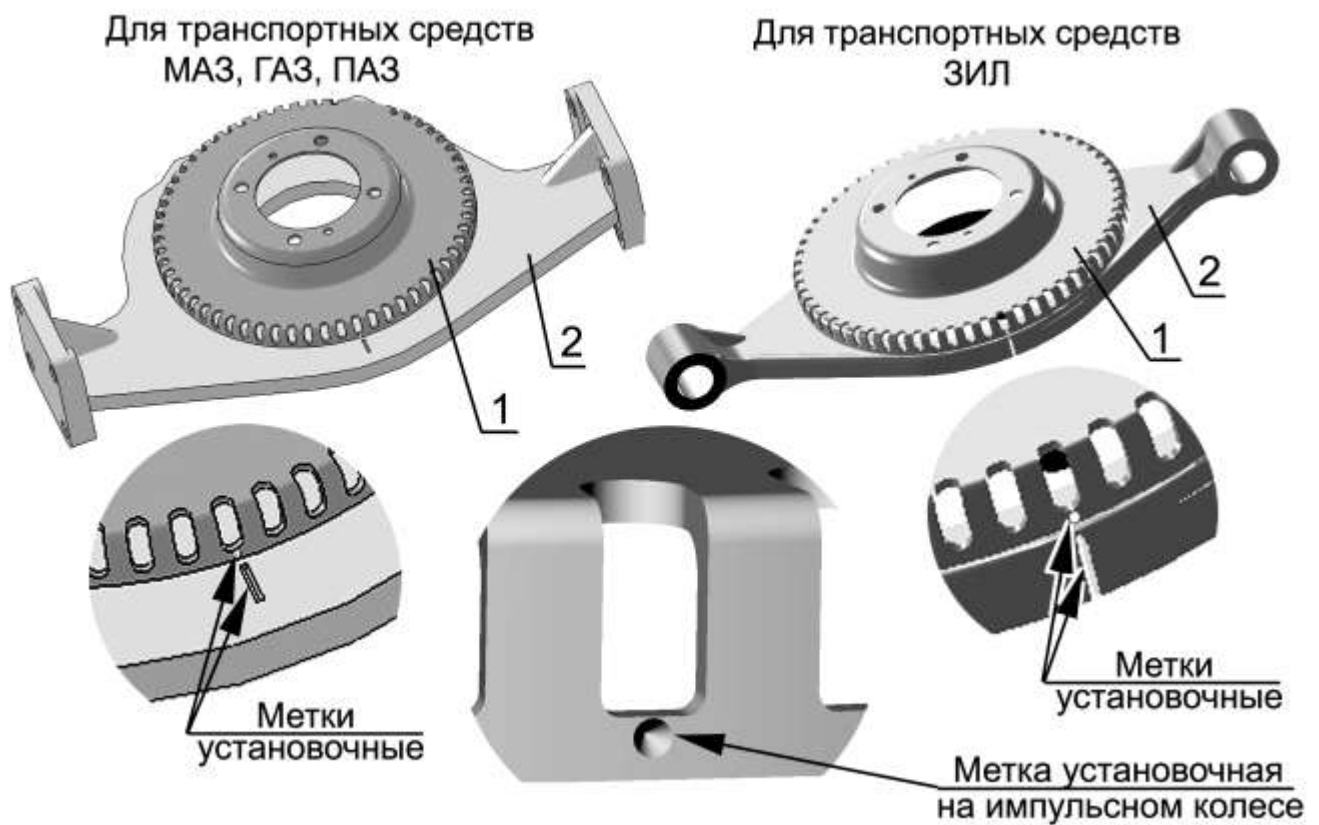
Рисунок 3а – Метки установочные.
