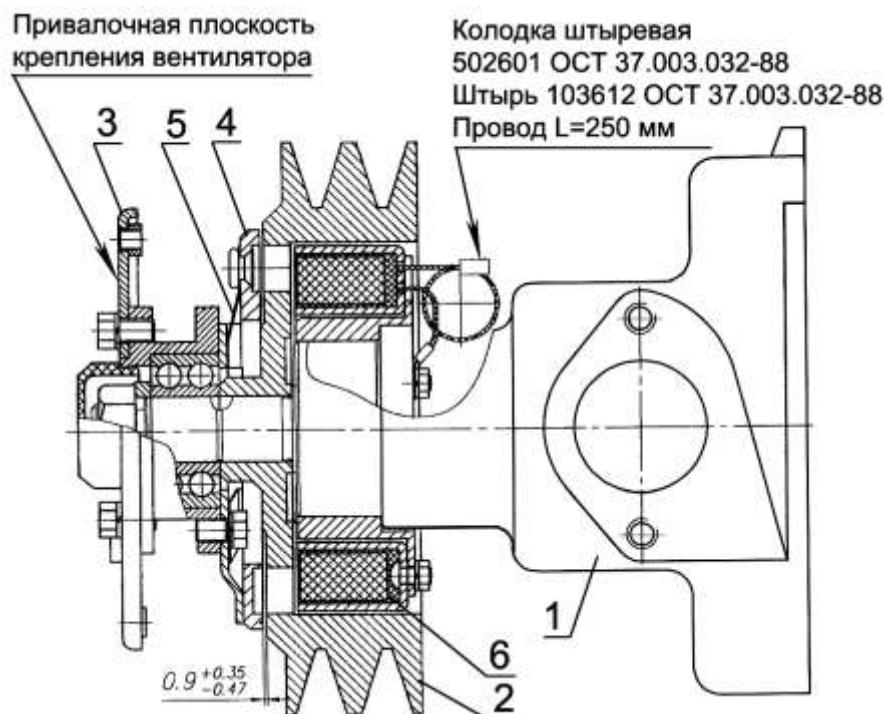
Рисунок 13 – Установка вентилятора
