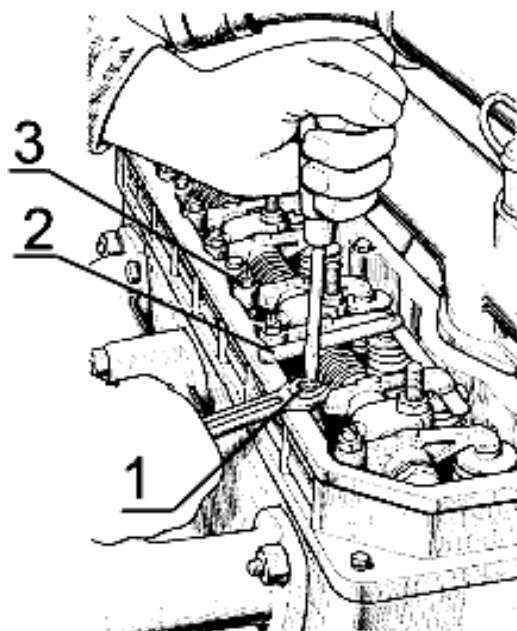
Рисунок 23 - Регулировка зазора в клапанах.
