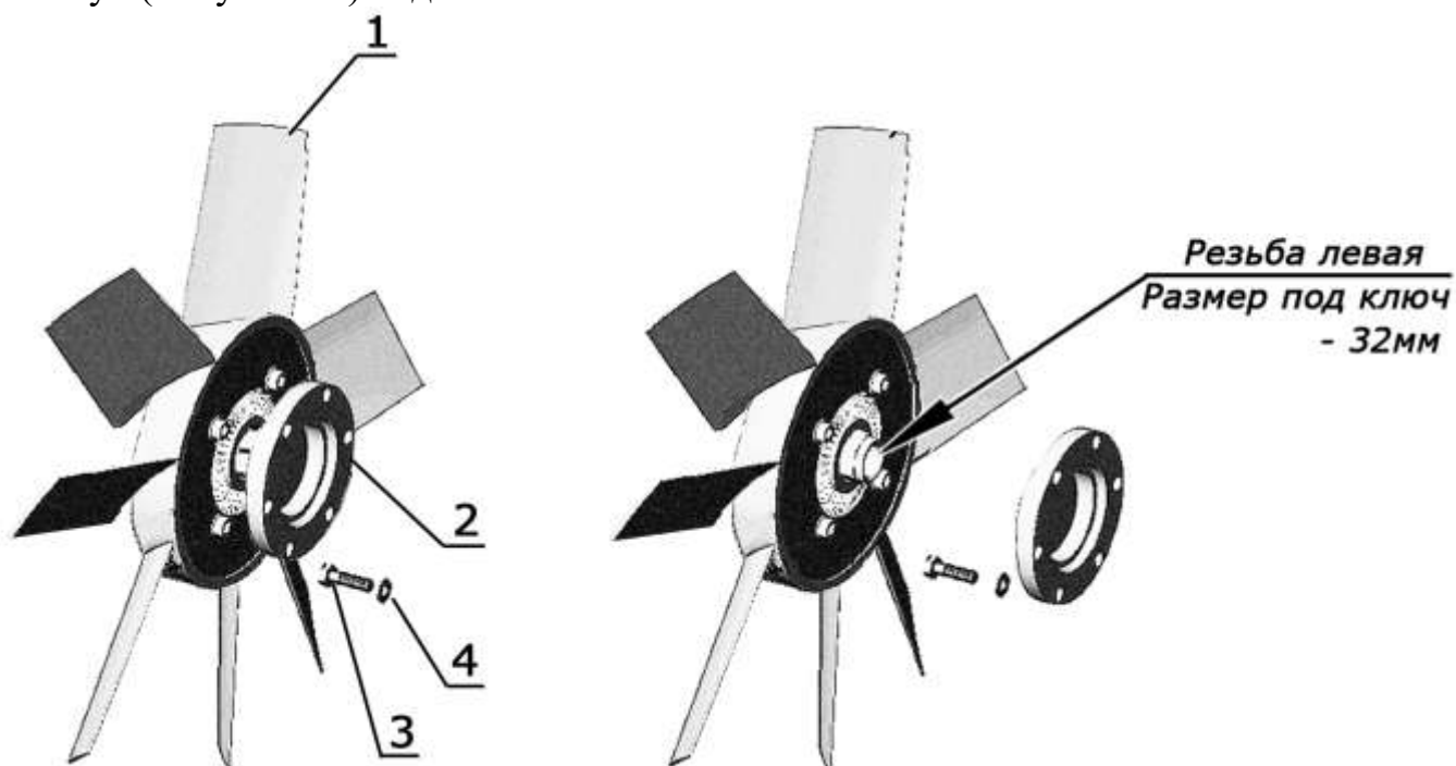
Рисунок 27б – Привод вентилятора
