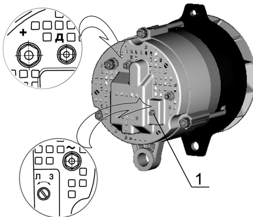
Рисунок 29 - Посезонная регулировка напряжения генератора
