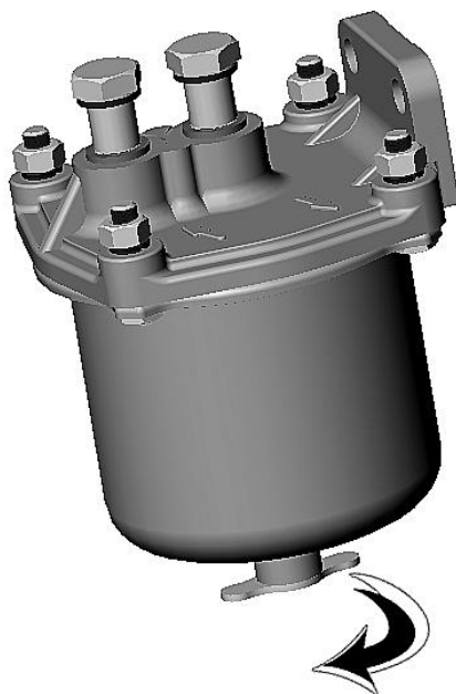
Рисунок 15– Слив отстоя из фильтра грубой очистки топлива.
