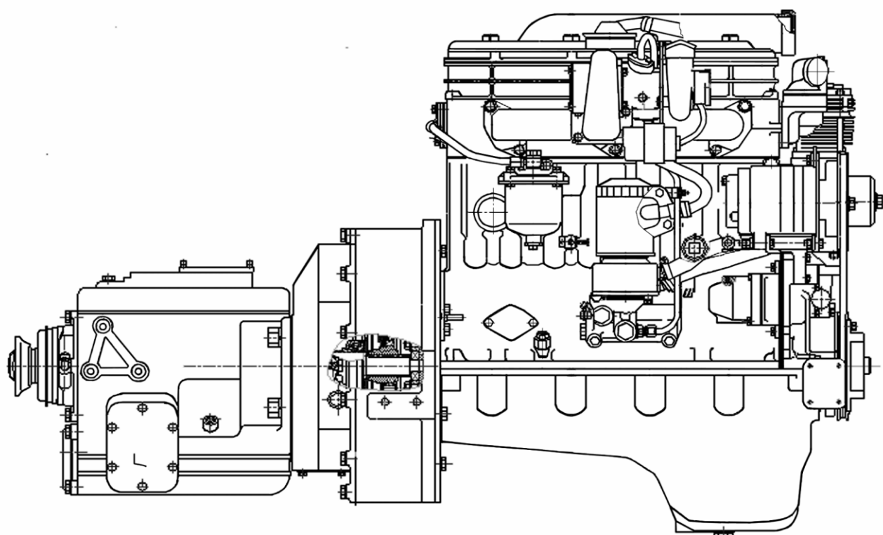
Вид слева
