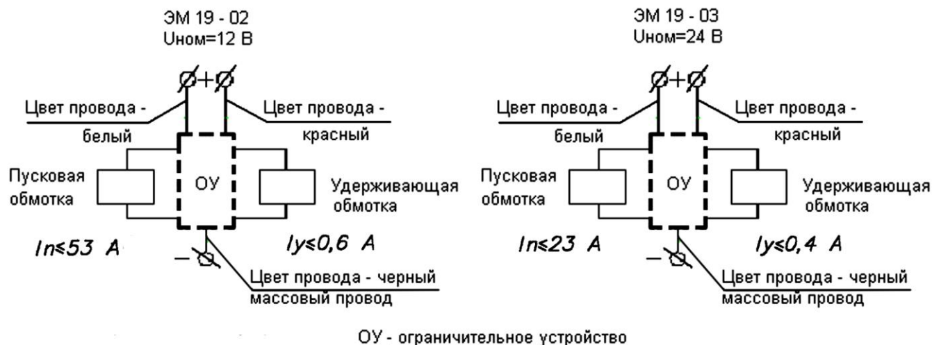
Рисунок 27 - Схема электрическая подключения электромагнита останова
