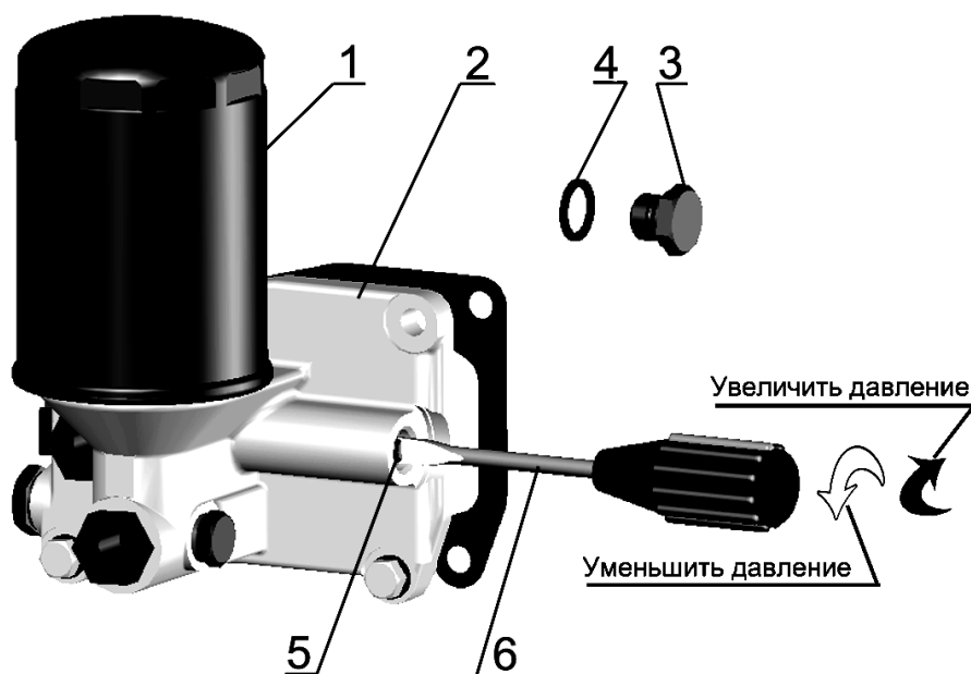
Рисунок 10а – Регулировка давления масла.
