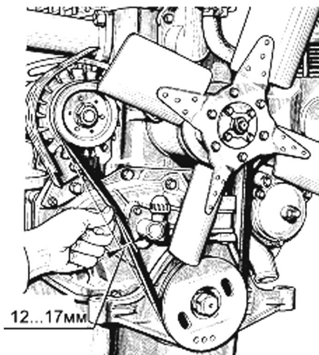
Рисунок 30 - Проверка натяжения ремня вентилятора.
