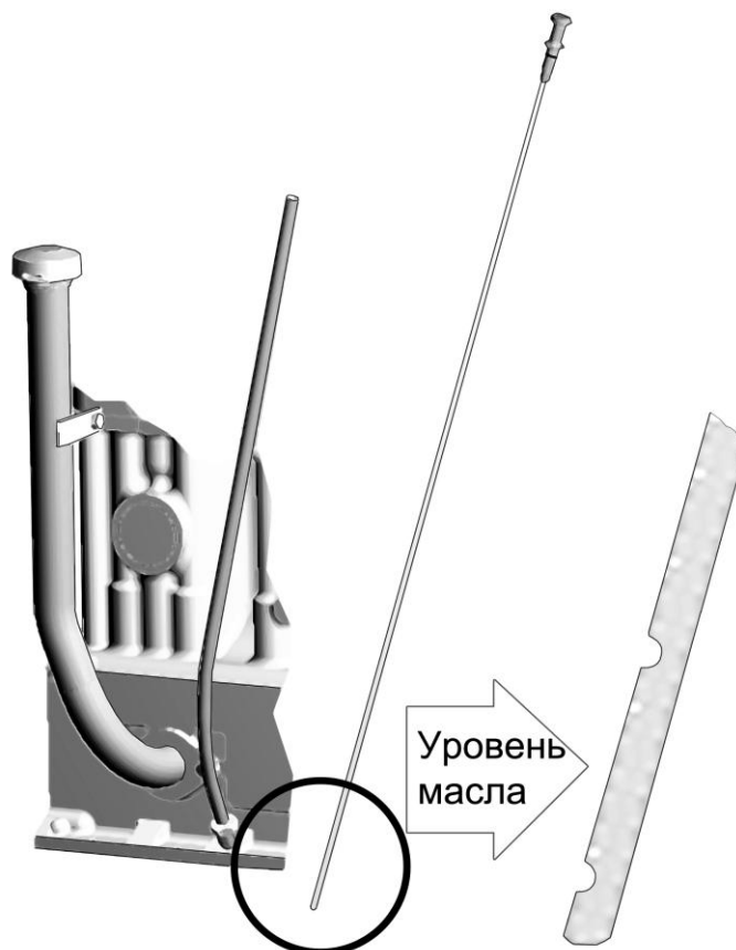
Рисунок 11- Проверка уровня масла в картере дизеля.
