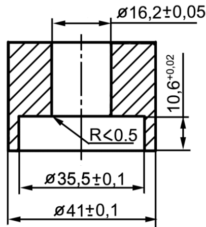
Рисунок 33- Оправка для запрессовки уплотнения водяного насоса (Основные конструктивные размеры)
