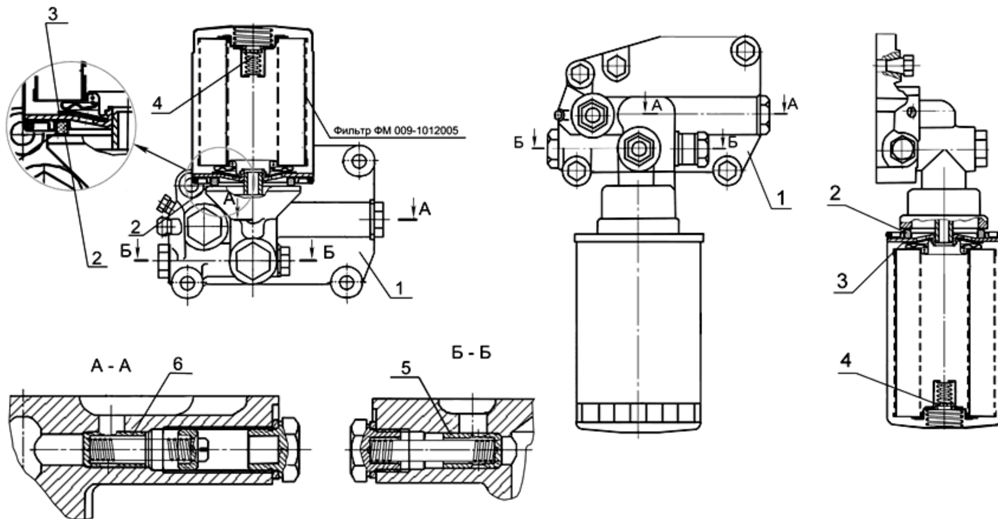
1 – корпус фильтра; 2 – прокладка; 3 – клапан противодренажный; 4 – клапан перепускной; 5 – клапан редукционный; 6 - клапан предохранительный. Рисунок 13 – Варианты установки масляного фильтра без ЖМТ на дизелях Д-245Е2
