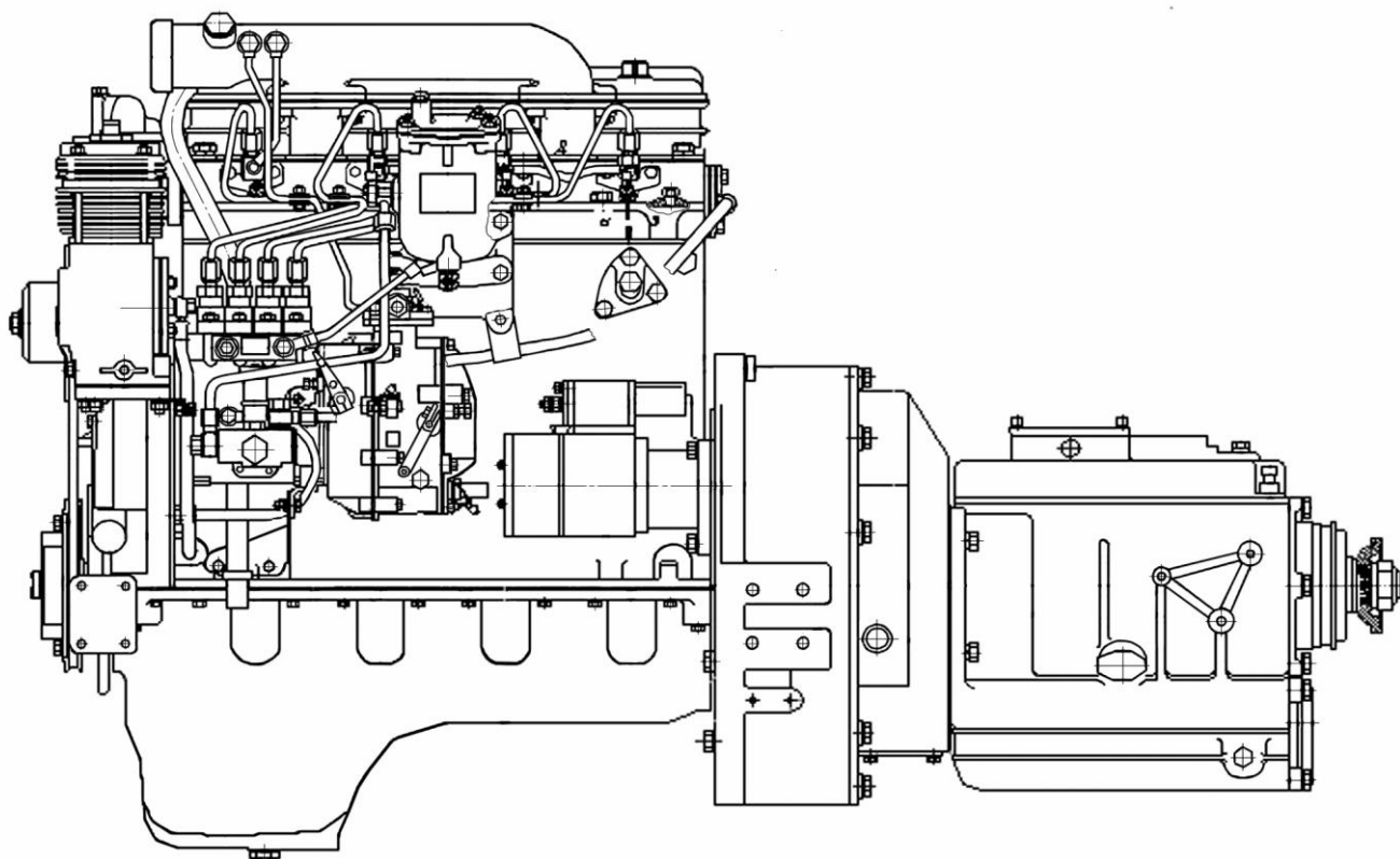
Вид слева
