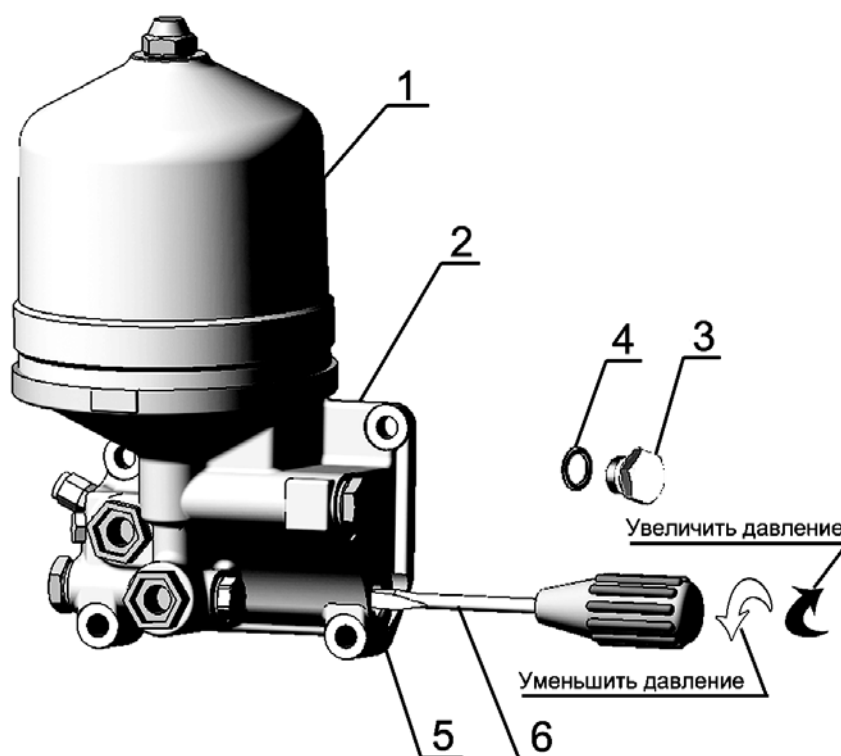
Рисунок 10в – Регулировка давления масла.
