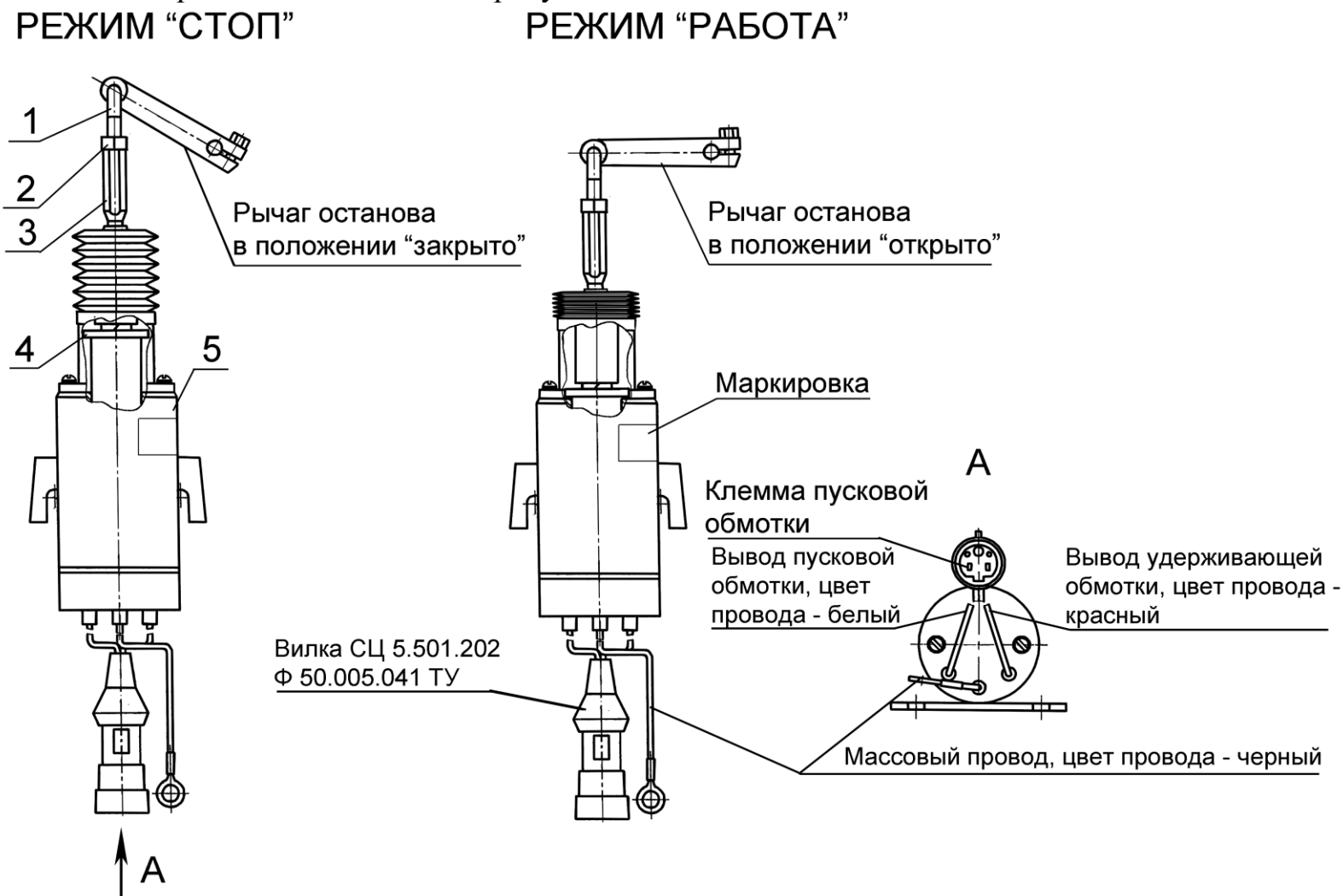
Рисунок 6 - Схема установки электромагнита останова
